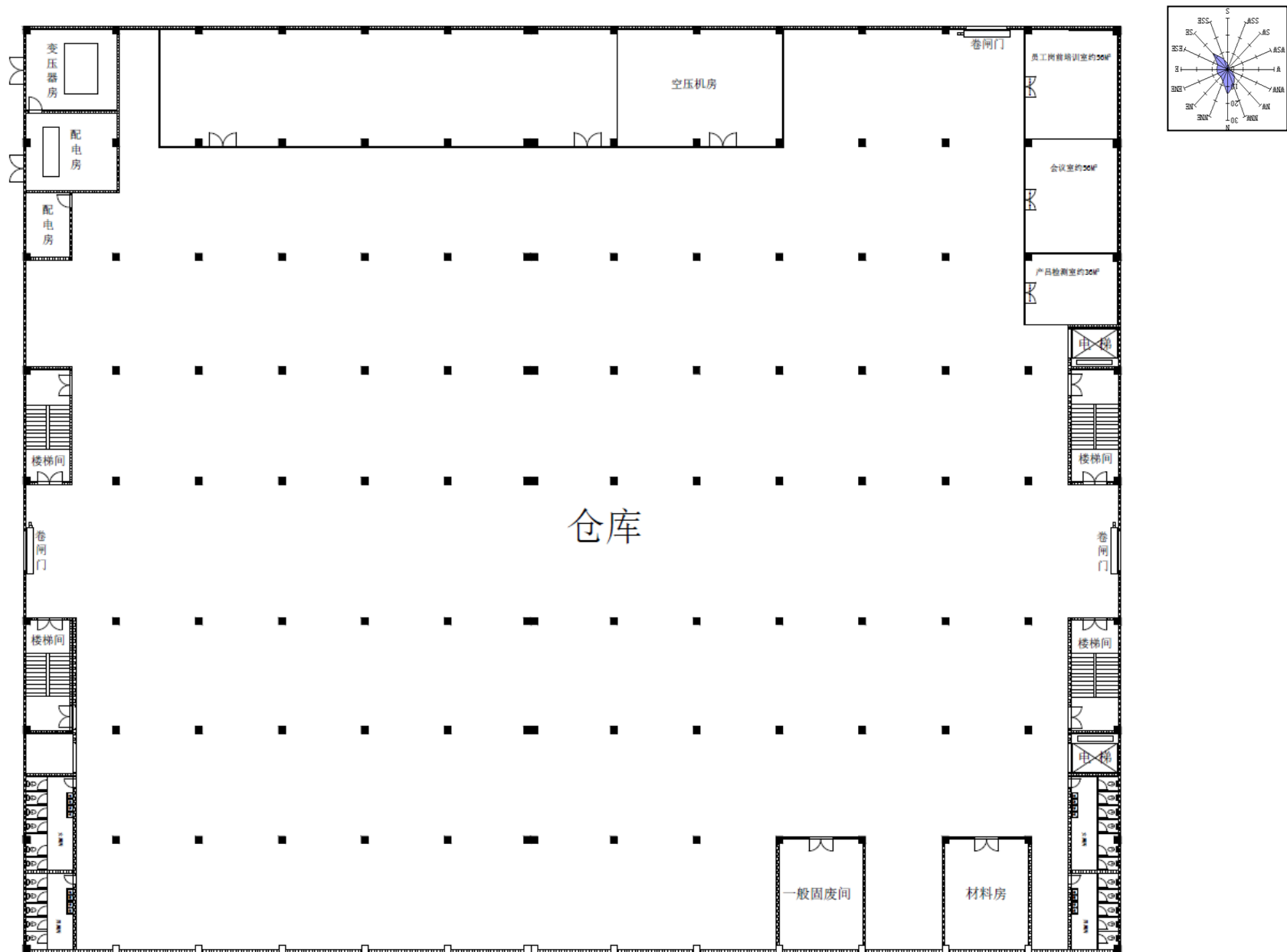
附图 5-2 项目生产厂房 1 楼平面布置图
