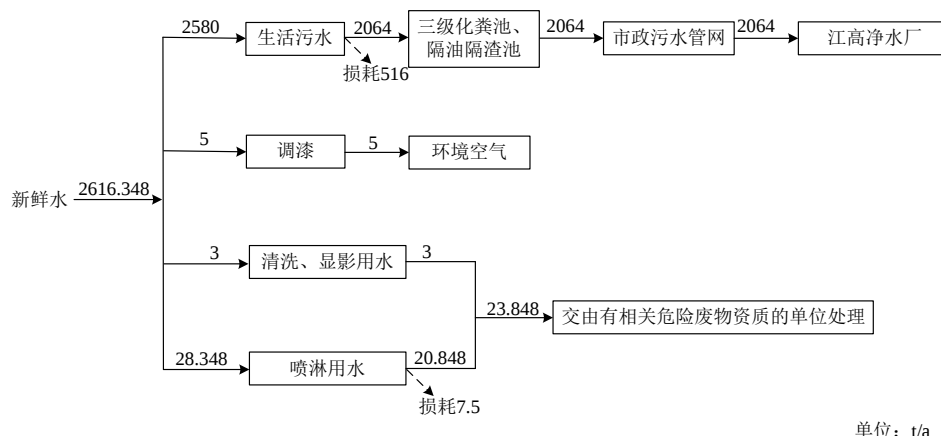
图 2-2 项目水平衡图
