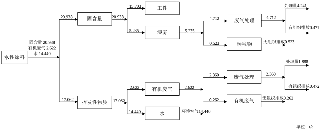
图 2-1 项目漆料平衡图
