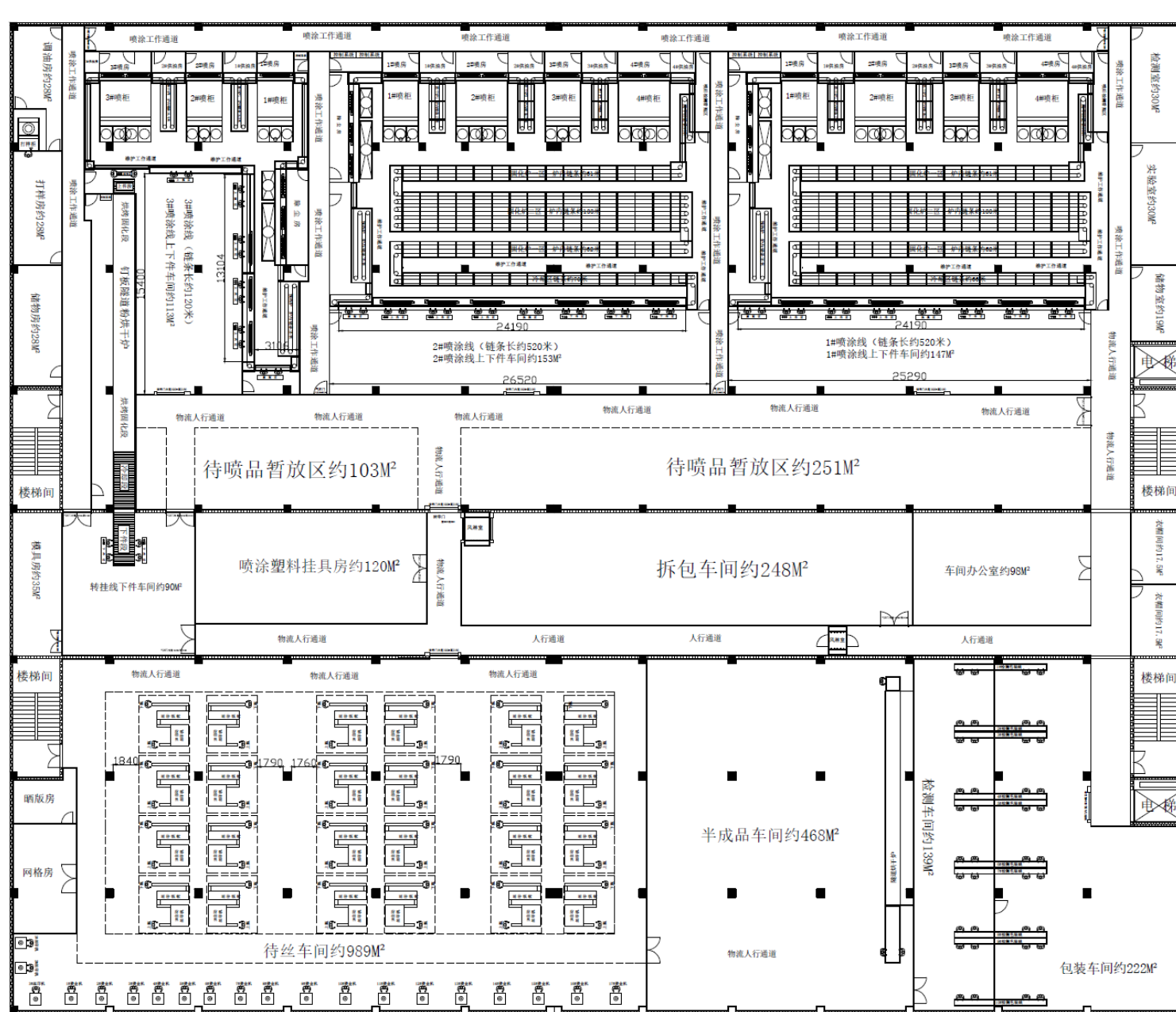
附图 5-3 项目生产厂房 2 楼平面布置图
