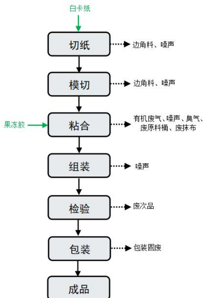
图 2-3 化妆品精装盒生产工艺流程及产污环节图
