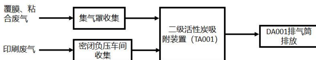
图 4-2 废气处理工艺图
