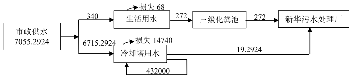
图 2-1 全厂水平衡图（单位：m 3 /a）
