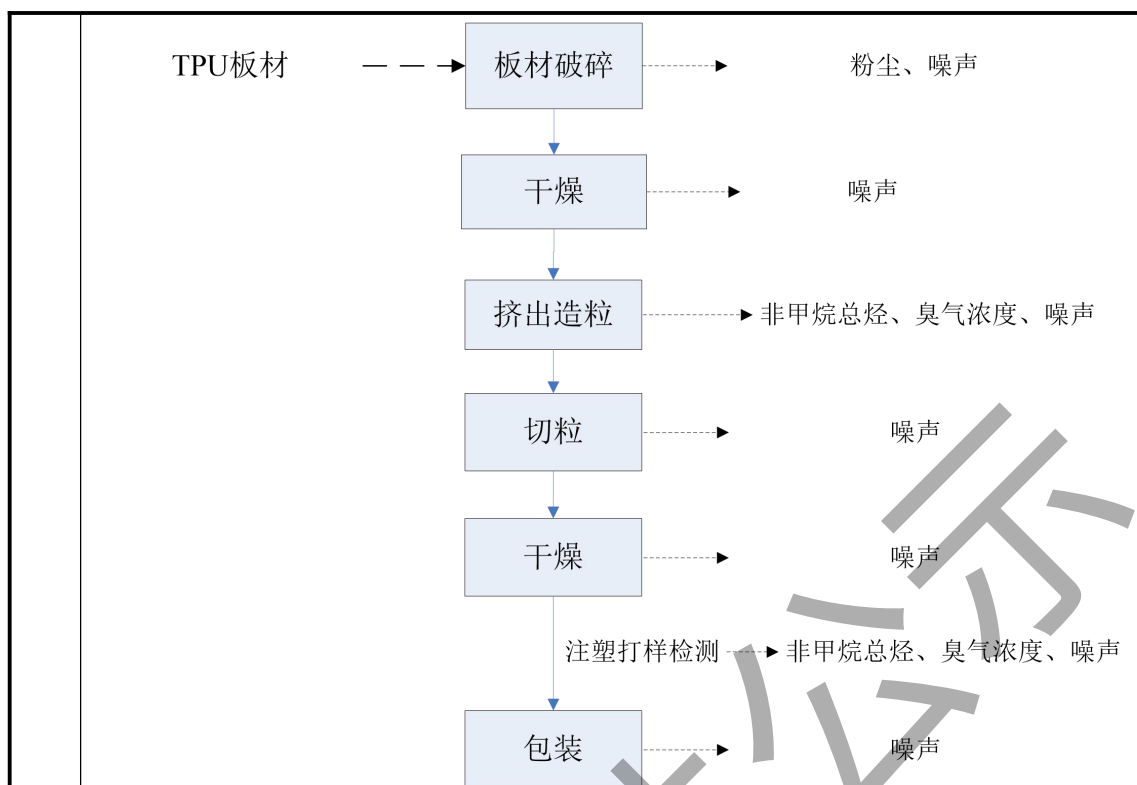
图 2-2 TPU塑料粒生产工艺流程图
