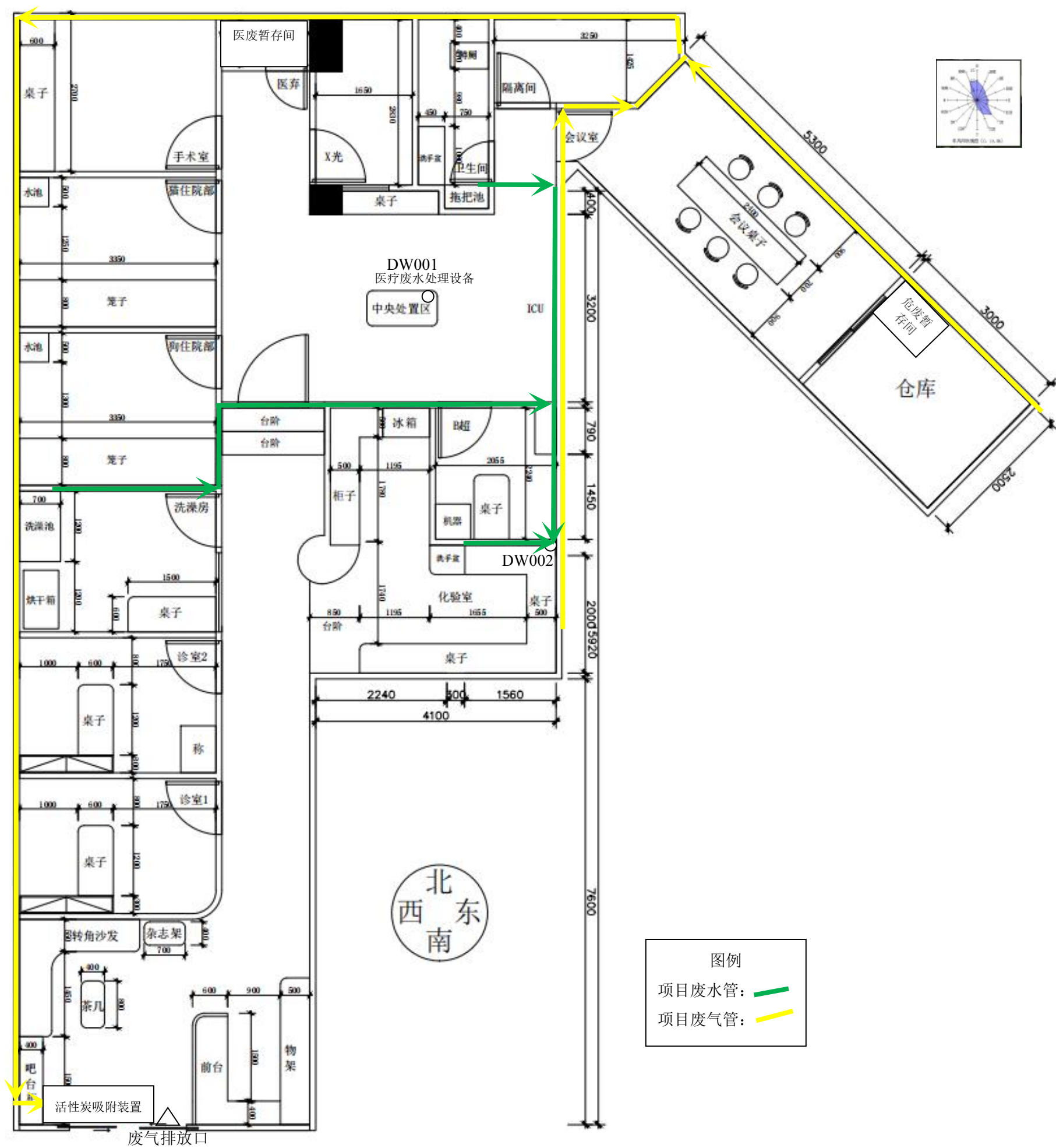
附图2 建设项目平面布置图 (1:500)
