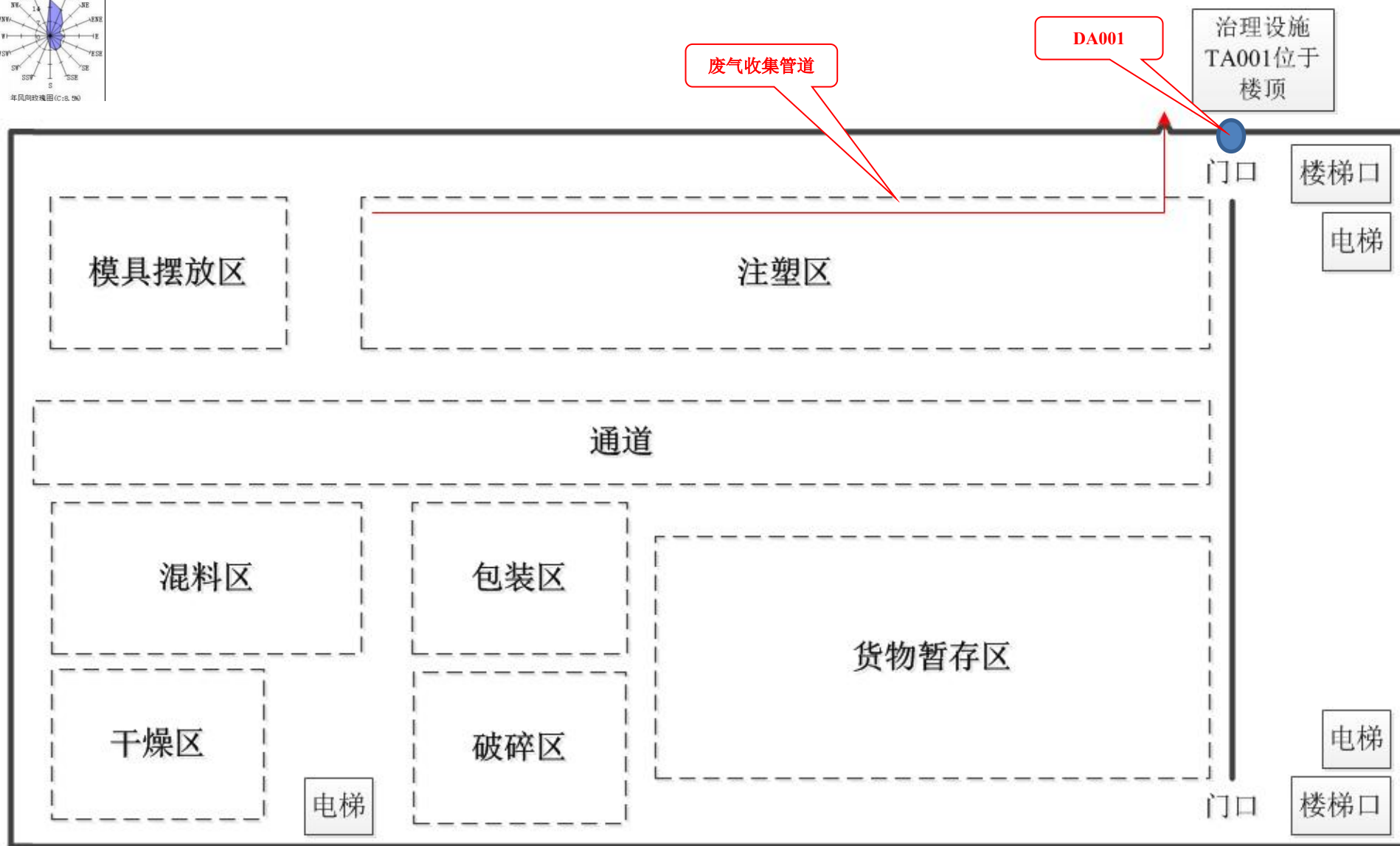
附图 4 建设项目 1F 平面布置图
