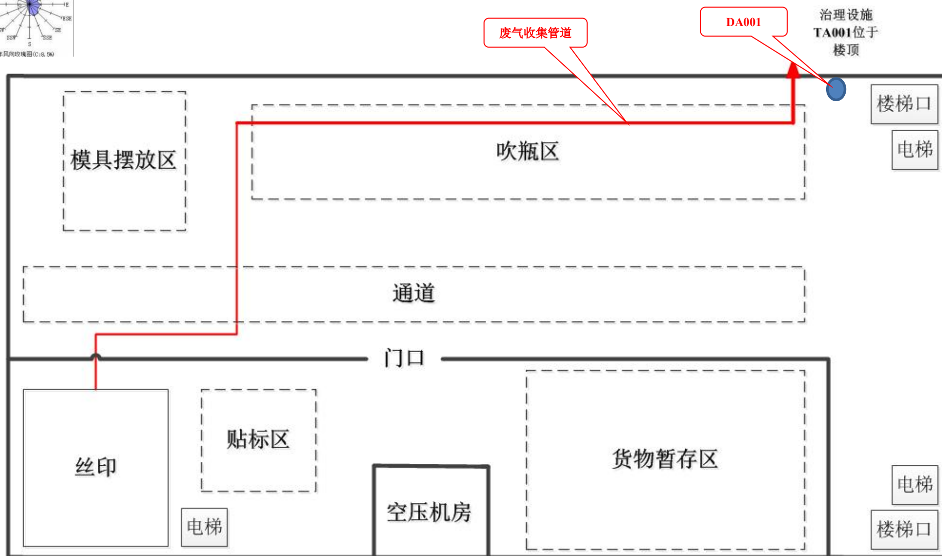
附图 6 建设项目 3F 平面布置图
