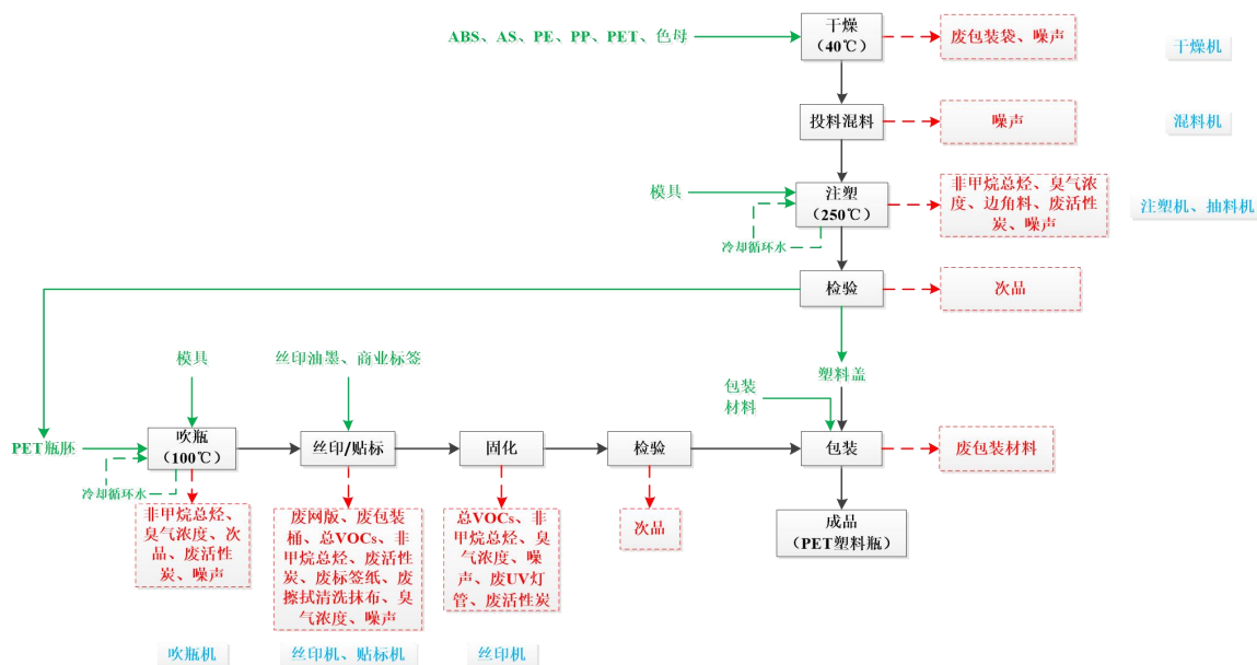
图 2-3 本项目 PET 塑料瓶生产工艺流程及产污环节图
