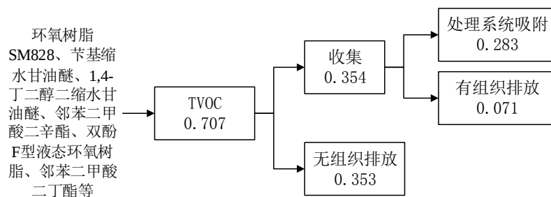
图 2-1 总 VOCs 平衡图（单位：t/a）
