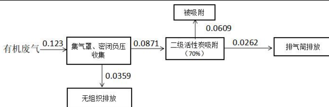
图 4-1 项目有机废气平衡图 (t/a)
