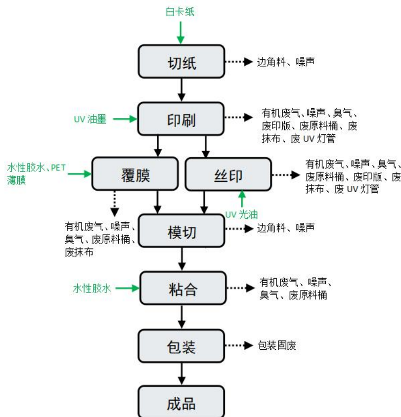
图 2-2 彩盒生产工艺流程及产污环节图
