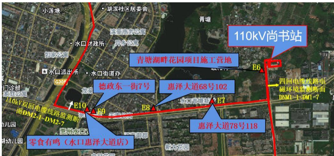
图 I-1 类比电缆线路监测布点图
