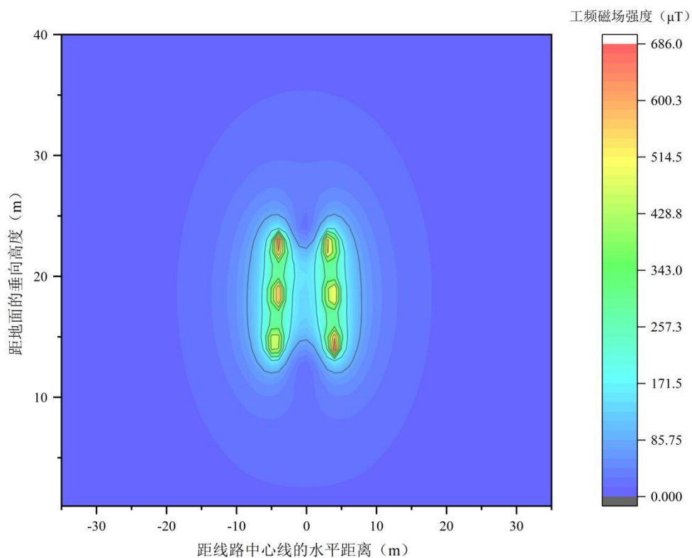
图 I-11 110kV 茶汉甲乙线工频磁场预测达标等值线图 (单位: μT)
