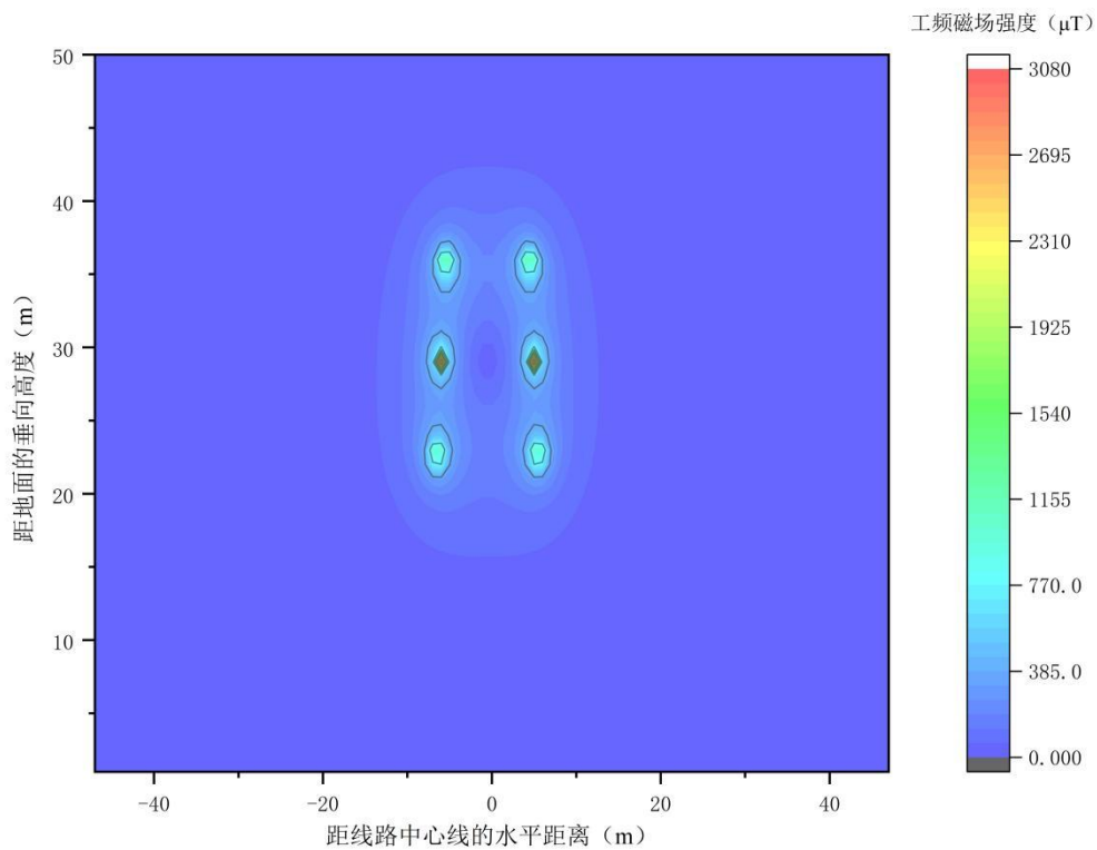
图 I-13 220kV 北麒甲乙线工频磁场预测达标等值线图 (单位: μT)
