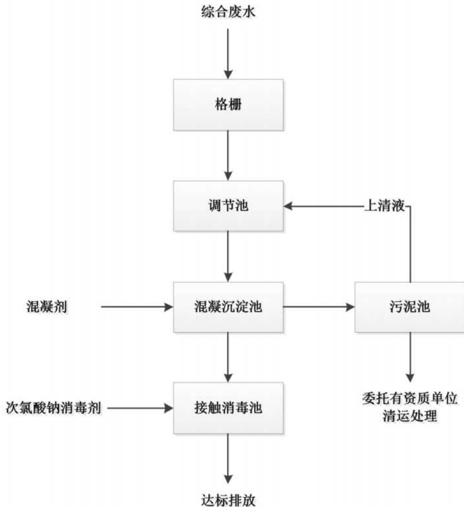
图7.1-1 项目自建污水处理站工艺流程图
