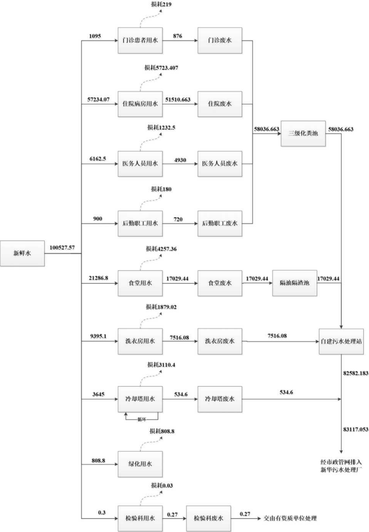
图 4.2-4 改扩建后整体项目年水平衡图 (单位 \text{m}^3/\text{a} )
