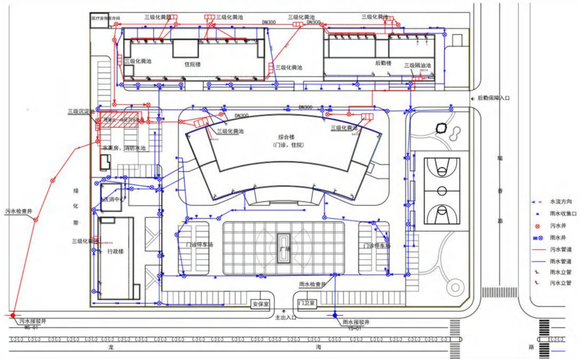
图 3.1-4 原有已审批项目雨污水管网分布图
