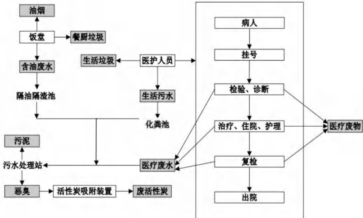
图 3.2-1 原有已审批项目运营期工作流程及产污环节图
