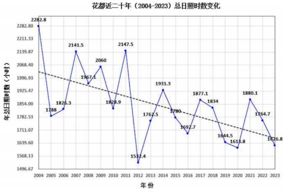
图 6.2-10 花都（2004-2023）年日照时长（单位：小时，虚线为趋势线）
