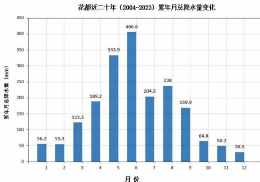
图 6.2-7 花都（2004-2023）累年月平均降水量（单位：毫米）
