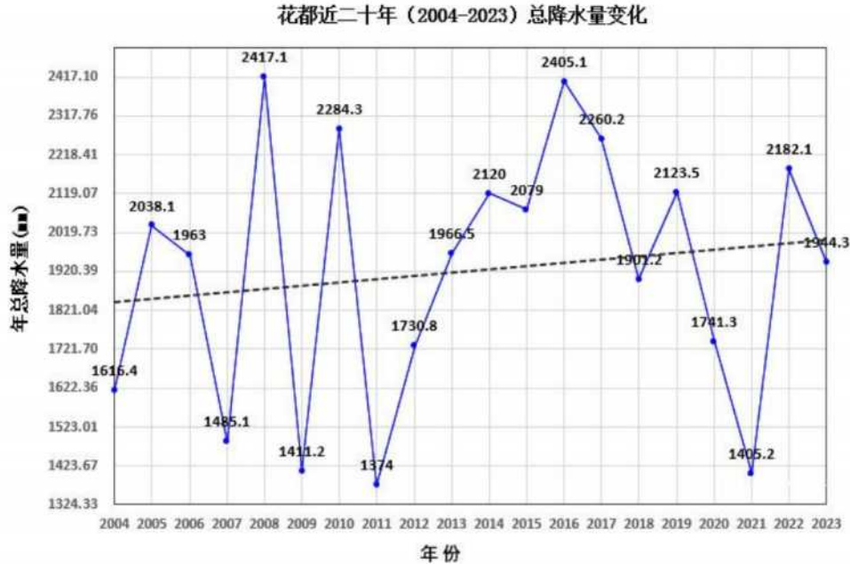
图 6.2-8 花都（2004-2023）年总降水量（单位：毫米，虚线为趋势线）
