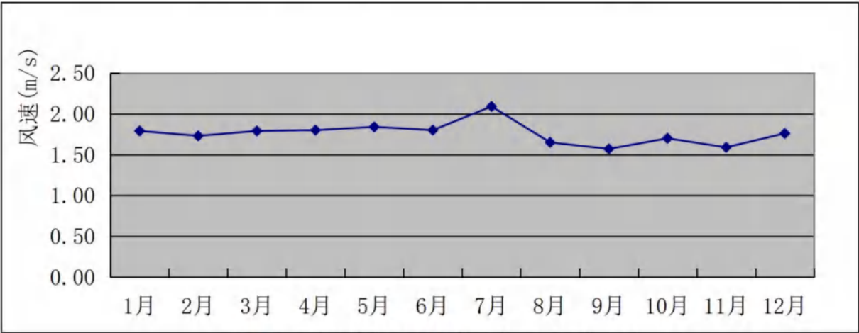
图 6.2-14 花都气象站 2023 年平均风速月变化图
