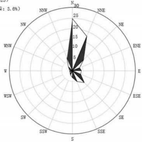
花都近二十年累年2月风向频率统计图
