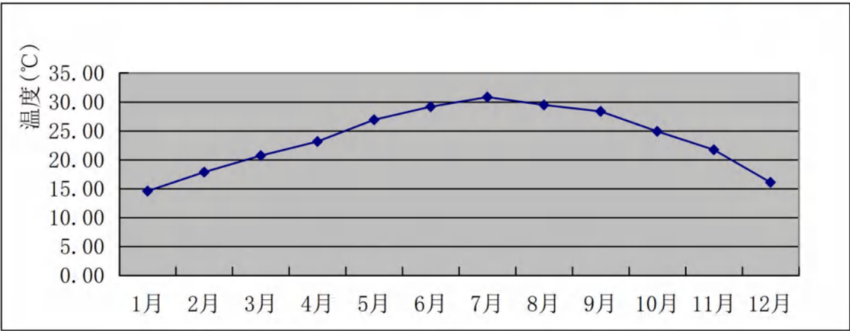
图 6.2-13 花都气象站 2023 年平均温度变化图
