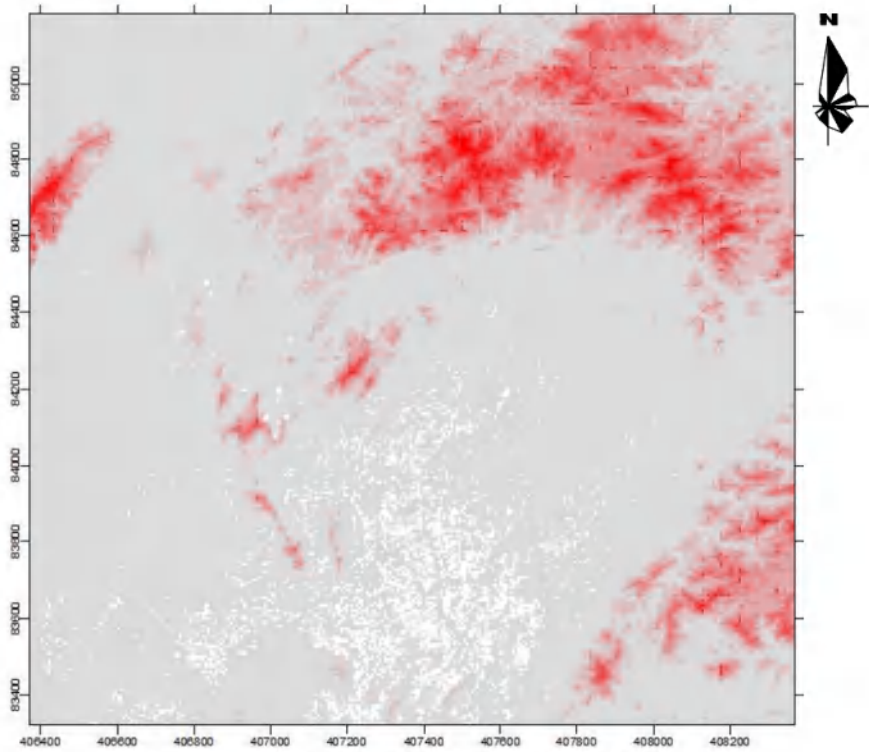
图 2.5-1 项目所在区域地形等高线示意图
