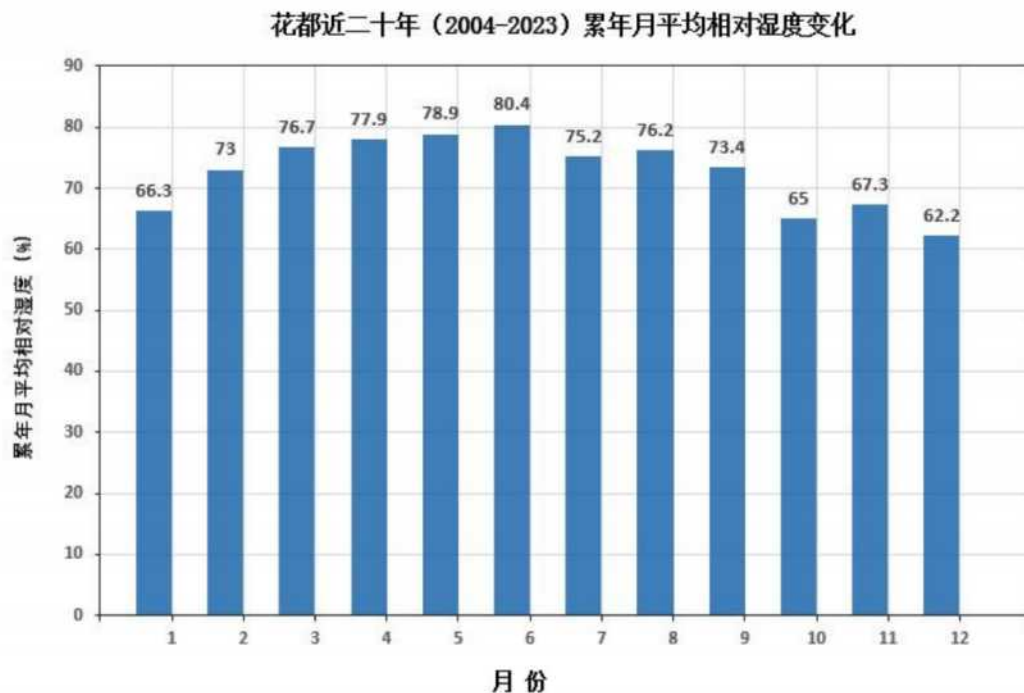
图 6.2-11 花都（2004-2023）累年月平均相对湿度（纵轴为百分比）
