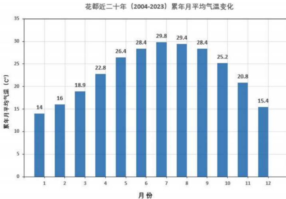
图 6.2-5 花都（2004-2023）累年月平均气温（单位：℃）
