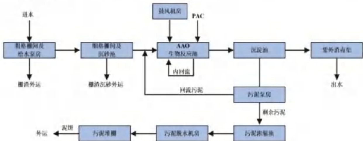
图 6.2-1 新华污水处理厂三期工程工艺流程简图
