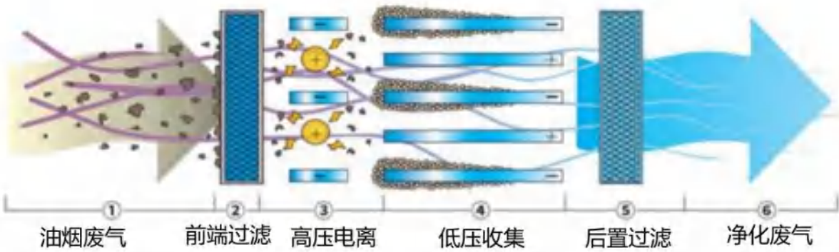
图 7.1-2 静电油烟净化器原理图
