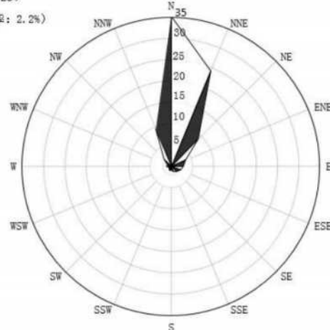
图 6.2-3 花都 (2004-2023) 累年月风向玫瑰图
