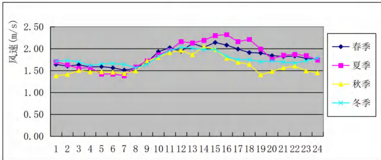
图 6.2-15 花都气象站 2023 年各季小时平均风速的日变化图
