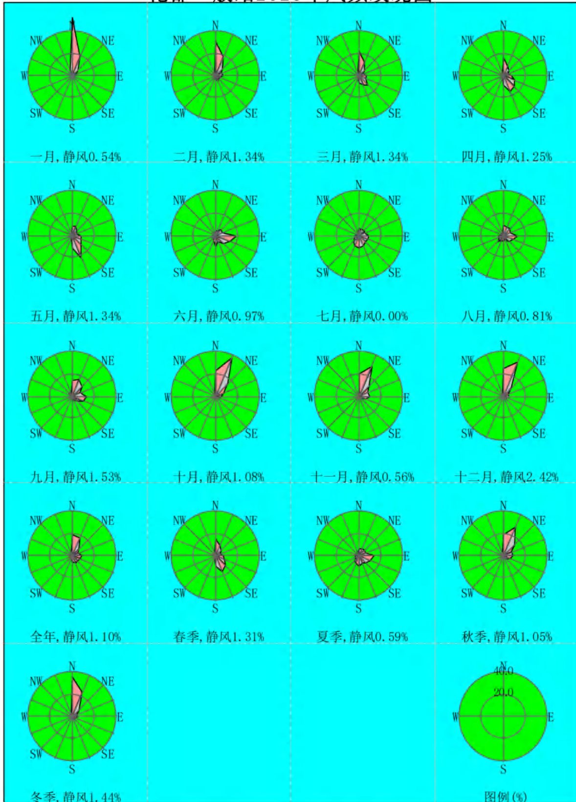
图 6.2-16 花都气象站 2023 年风频玫瑰图
