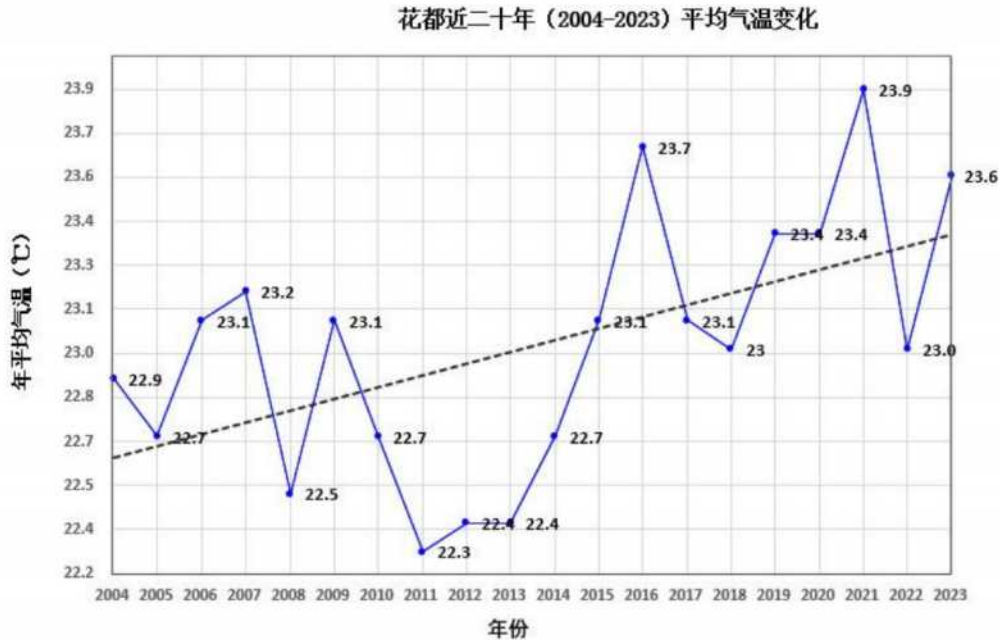
图 6.2-6 花都（2004-2023）年平均气温（单位：℃，虚线为趋势线）
