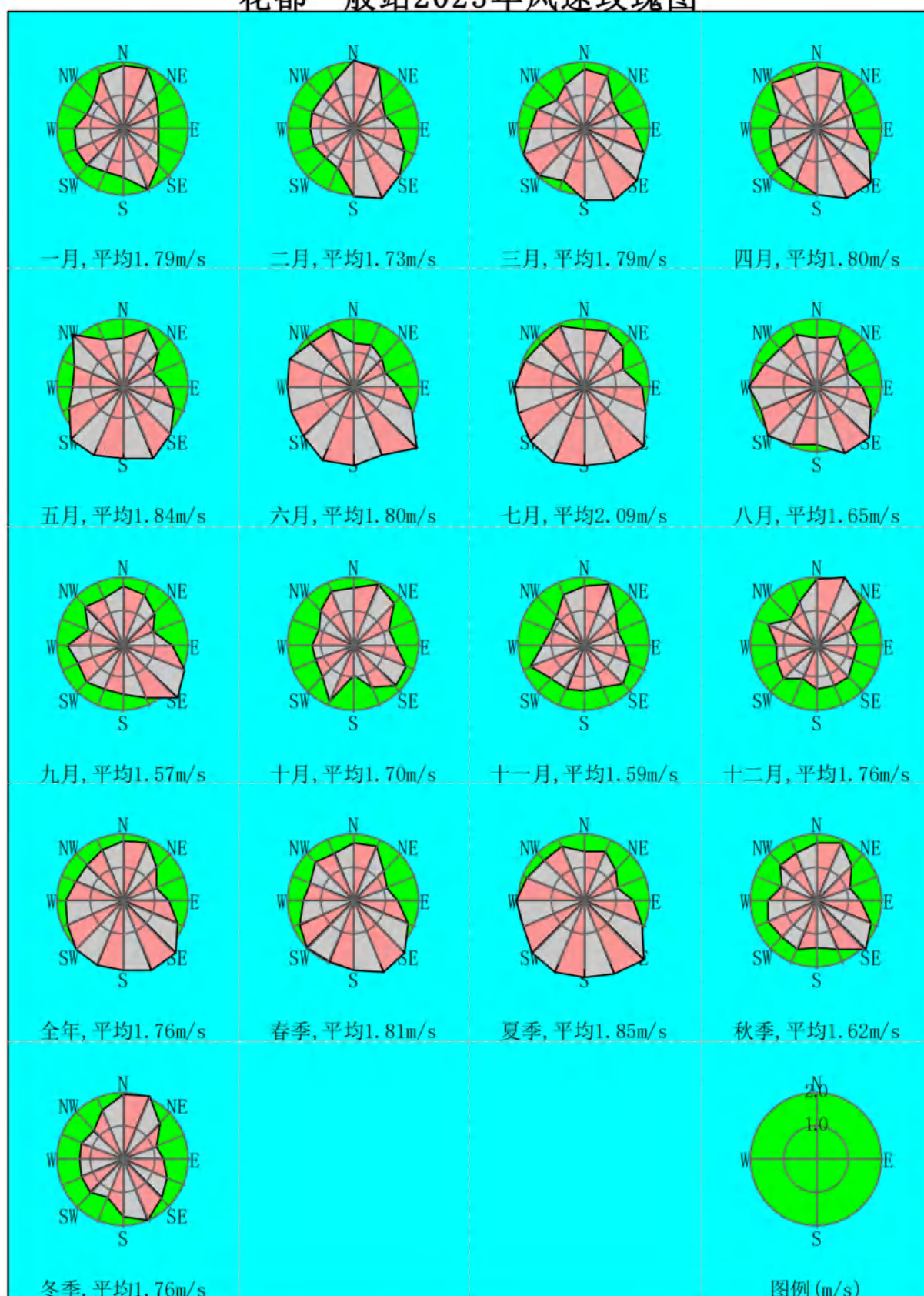
图 6.2-17 花都气象站 2023 年风速玫瑰图
