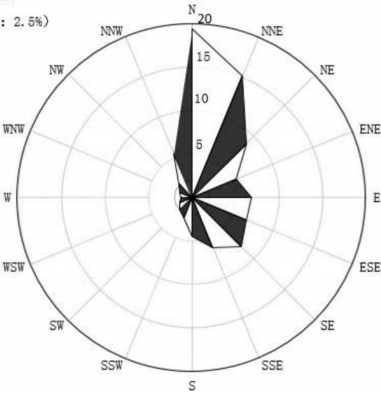
图 6.2-2 花都风向玫瑰图 (静风频率 2.5%)
