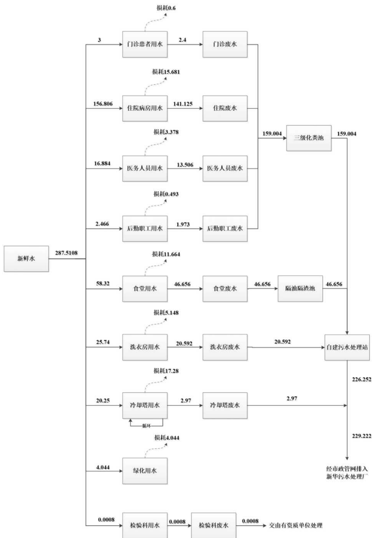
图 4.2-5 改扩建后整体项目最高日水平衡图（单位 m³/d）
