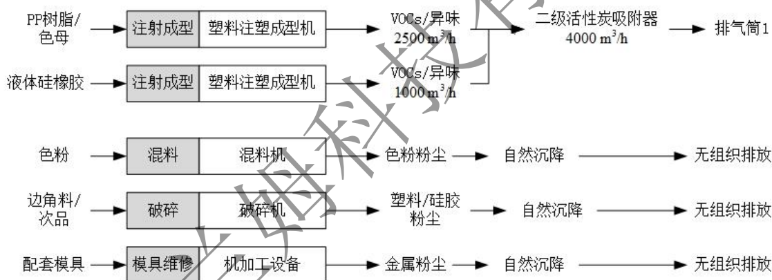
图 4-2 废气收集、治理和排放汇总示意图
