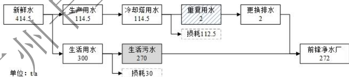
图 2-1 水平衡示意图
