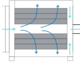
图 4-1 一级活性炭吸附装置示意图
