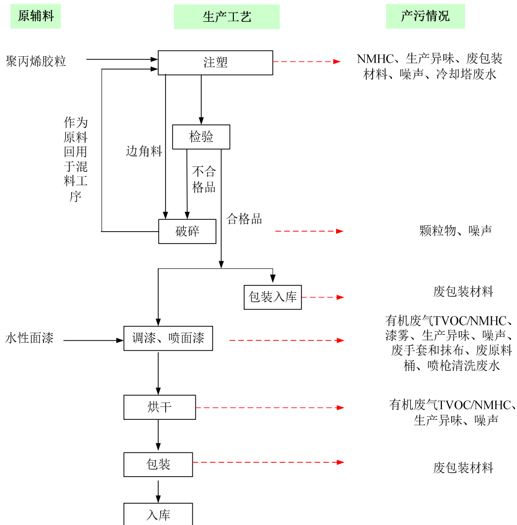
图 2-3 生产工艺流程及产污环节图
