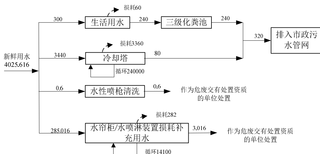
图 2-2 本项目水平衡图 (m³/a)
