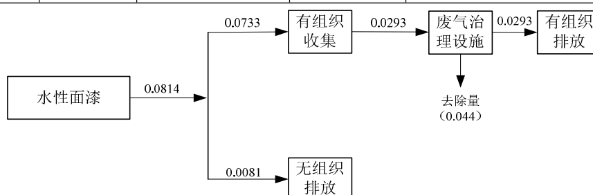
图 2-1 本项目 VOCs 平衡图 (t/a)
