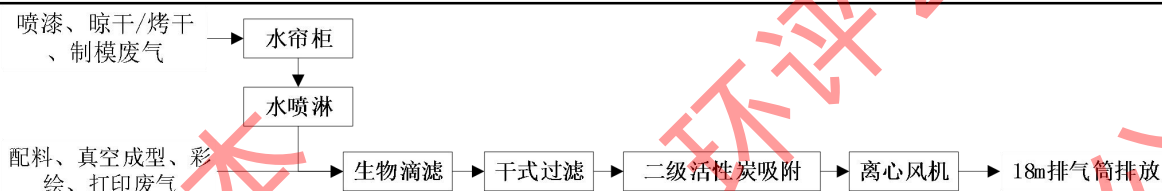
图 4-2 废气处理工艺流程图
