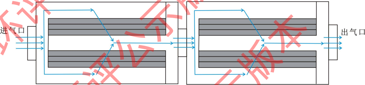
二级活性炭吸附装置工作示意图
