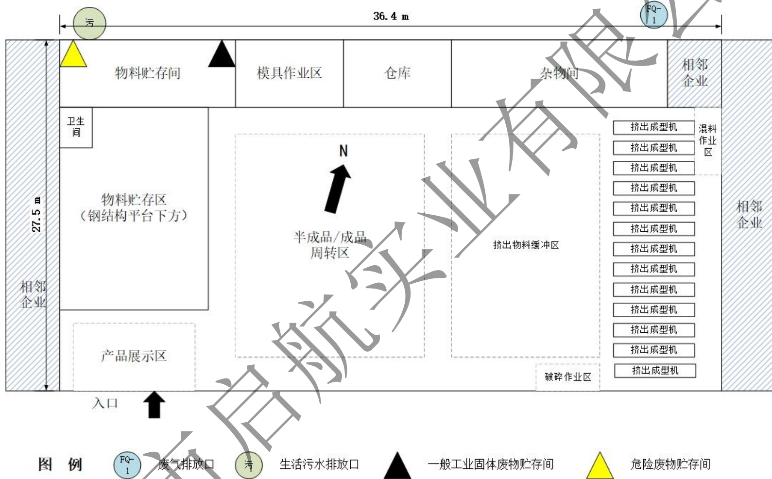
附图 3-1 平面布置图—地面层
