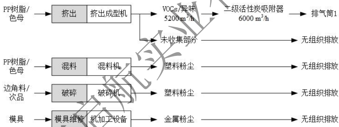
图 4-2 废气收集、治理和排放汇总示意图
