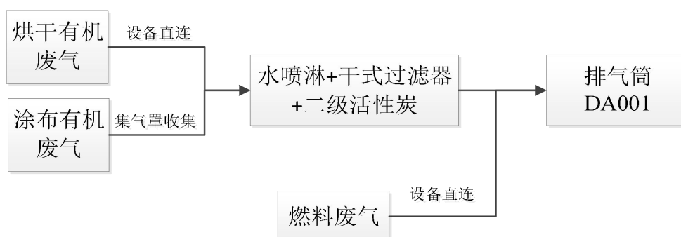
图 4-2 本项目废气处理工艺流程示意图
