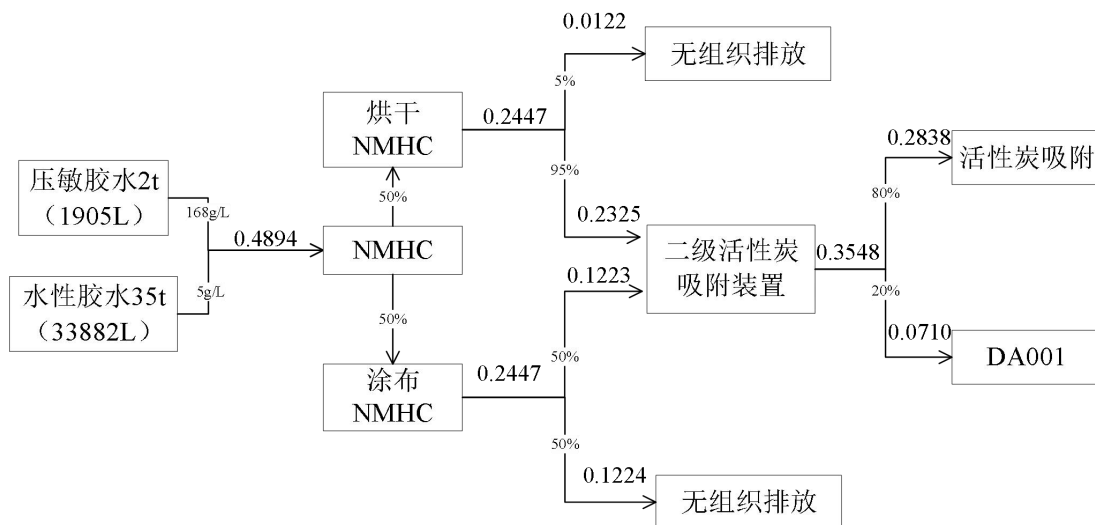
图 4-1 有机废气平衡图 单位:t/a
