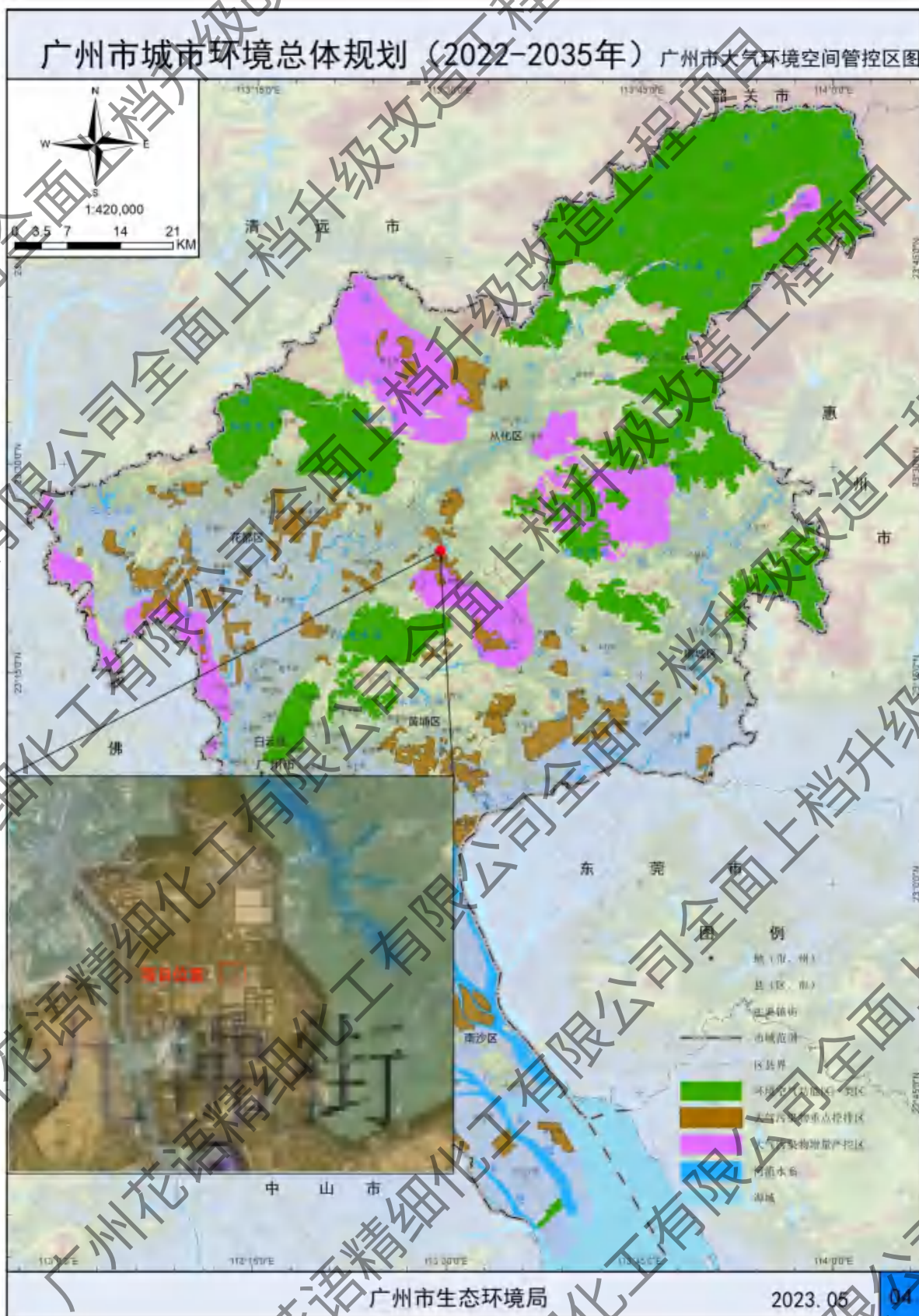
图1.4-4 广州市大气环境空间管控区图
