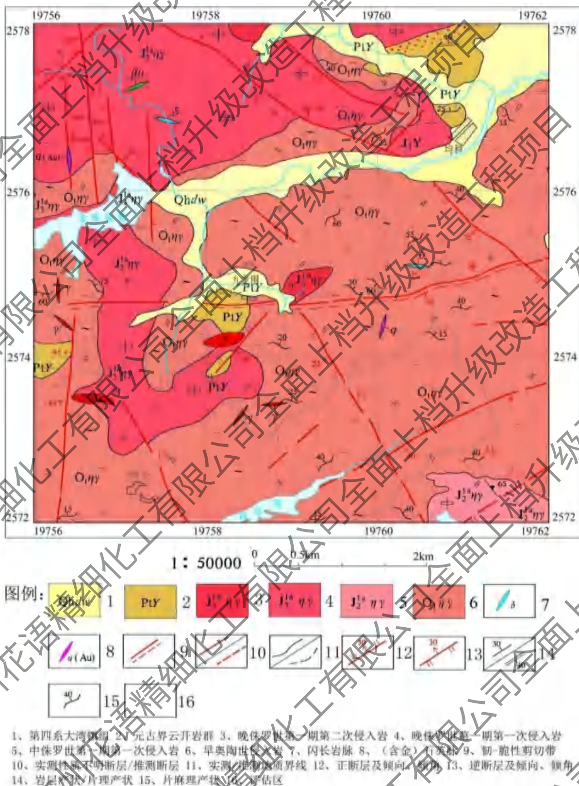
图 5.2-2 区域地质图
