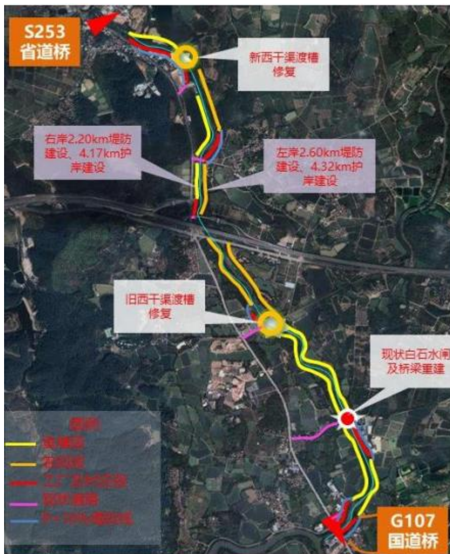
图 2-1 白坭河国泰水堤防达标整治工程布置图
