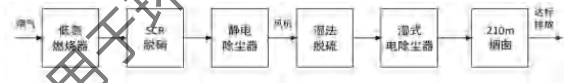
图 3.4.2-1 锅炉烟气治理工艺流程
