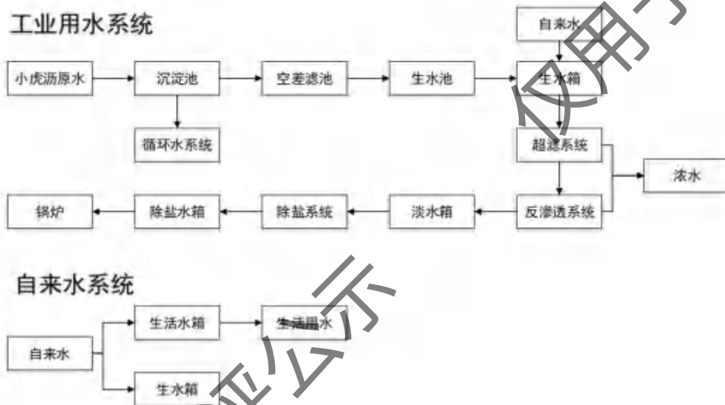
图 3.2.5-1 现有项目供水工艺流程图
