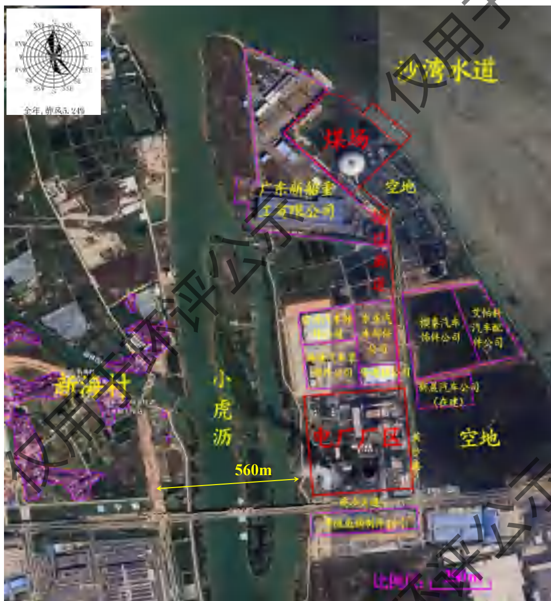
图 3.2.1-1 现有项目四至图
