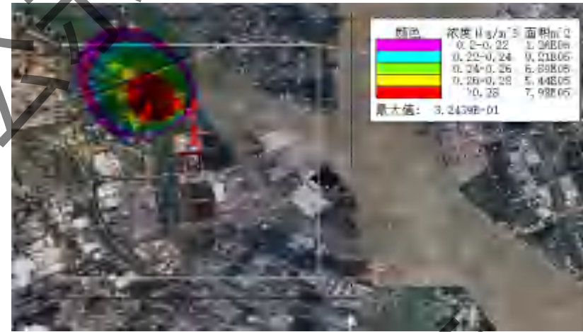
NO 2 年平均质量浓度
