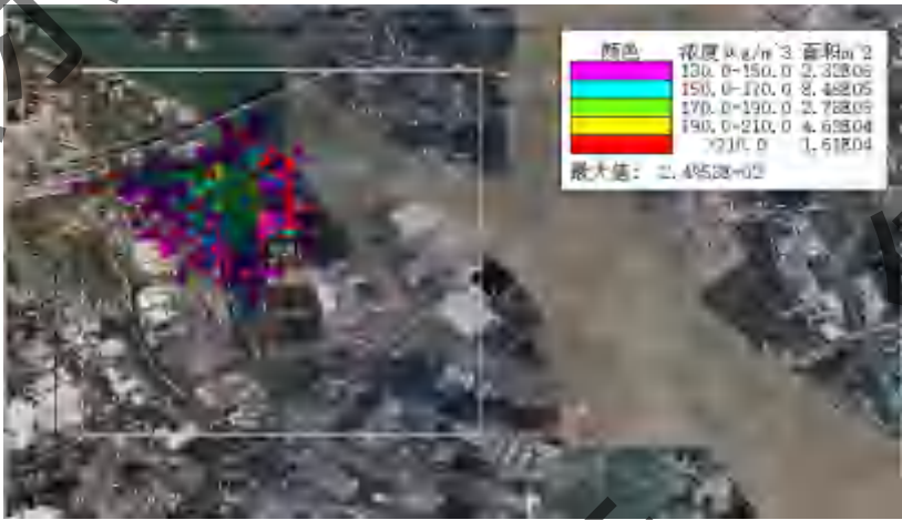
TSP 叠加后年平均质量浓度
