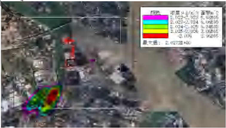
氯化氢叠加后日平均质量浓度
