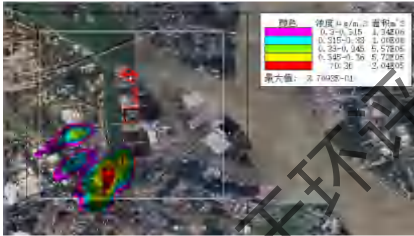
氟化物小时平均质量浓度
