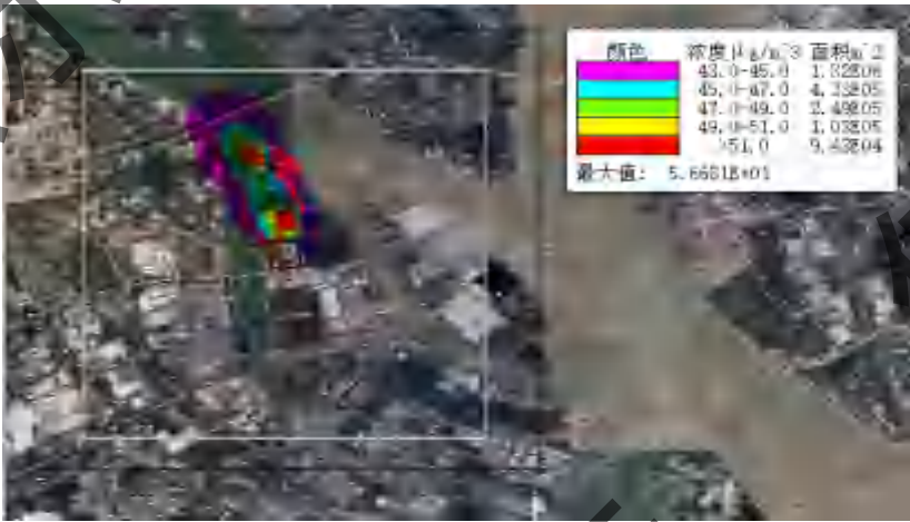
PM 10 叠加后年平均质量浓度
