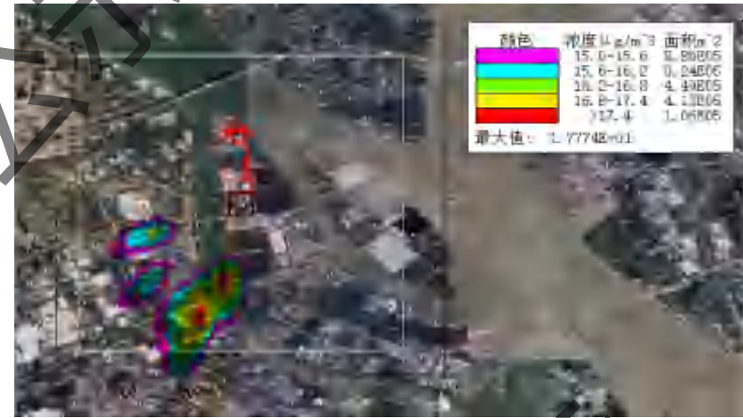
NO 2 小时平均质量浓度
