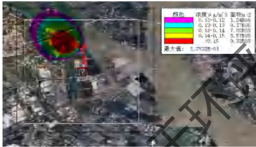
SO 2 年平均质量浓度
