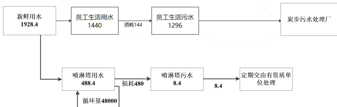
图 3 项目远期水平衡图 (单位: t/a)
