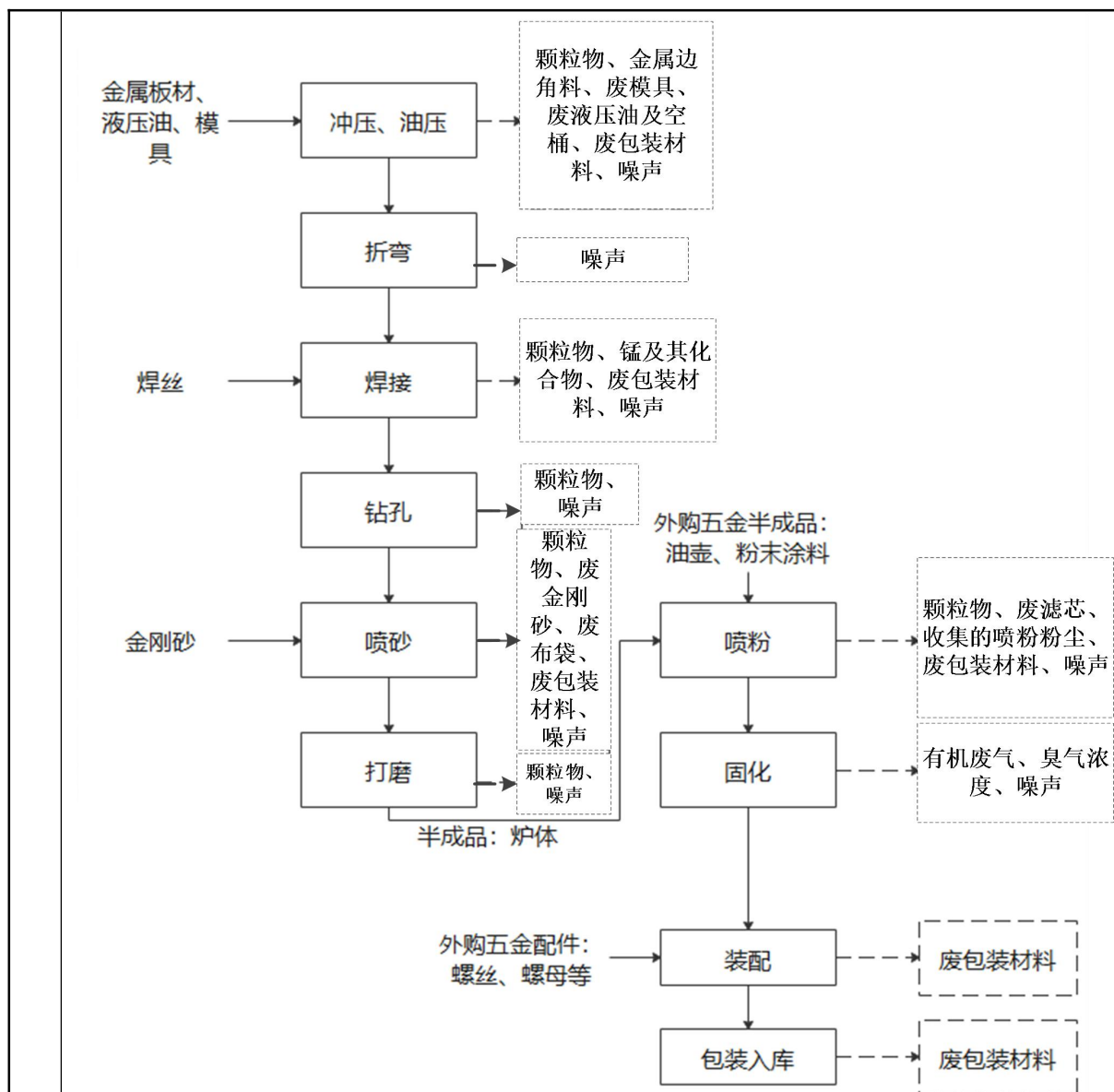
图 4 取暖炉生产工艺流程及产污环节图
