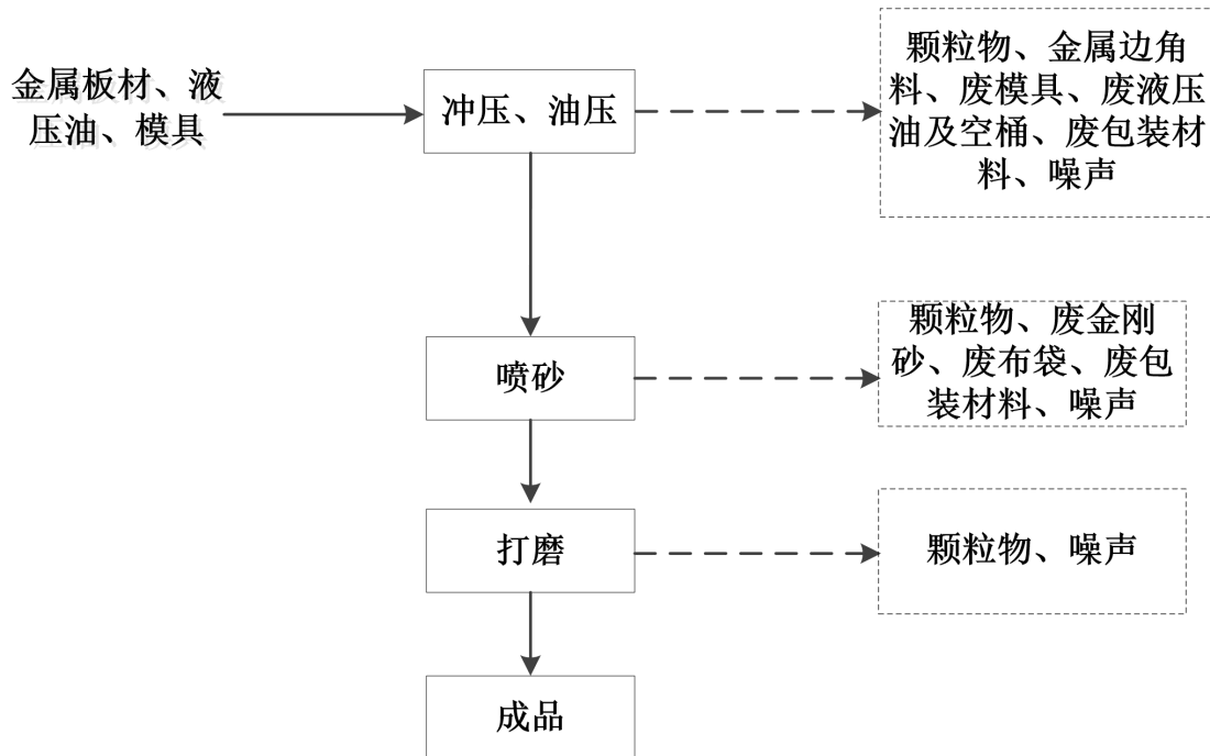
图 6 现有项目生产工艺流程及产污环节图
