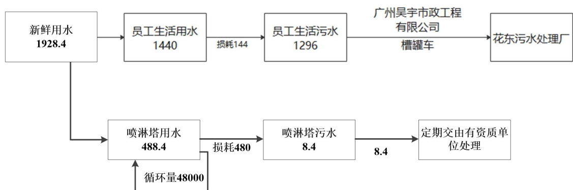
图 2 项目近期水平衡图 (单位: t/a)
