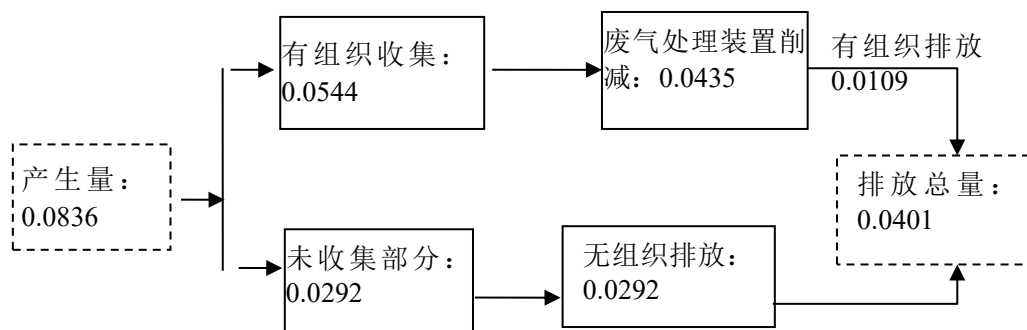
图1 项目TVOC、NMHC平衡图（单位：t/a）
