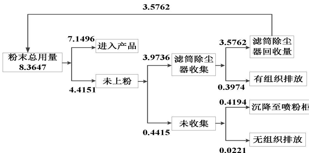
图 7 喷粉粉尘平衡图 (t/a)
