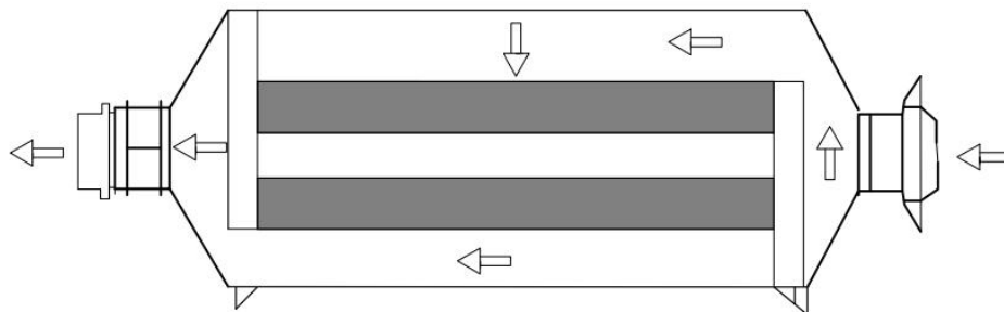
图 8 本项目活性炭箱设计图
