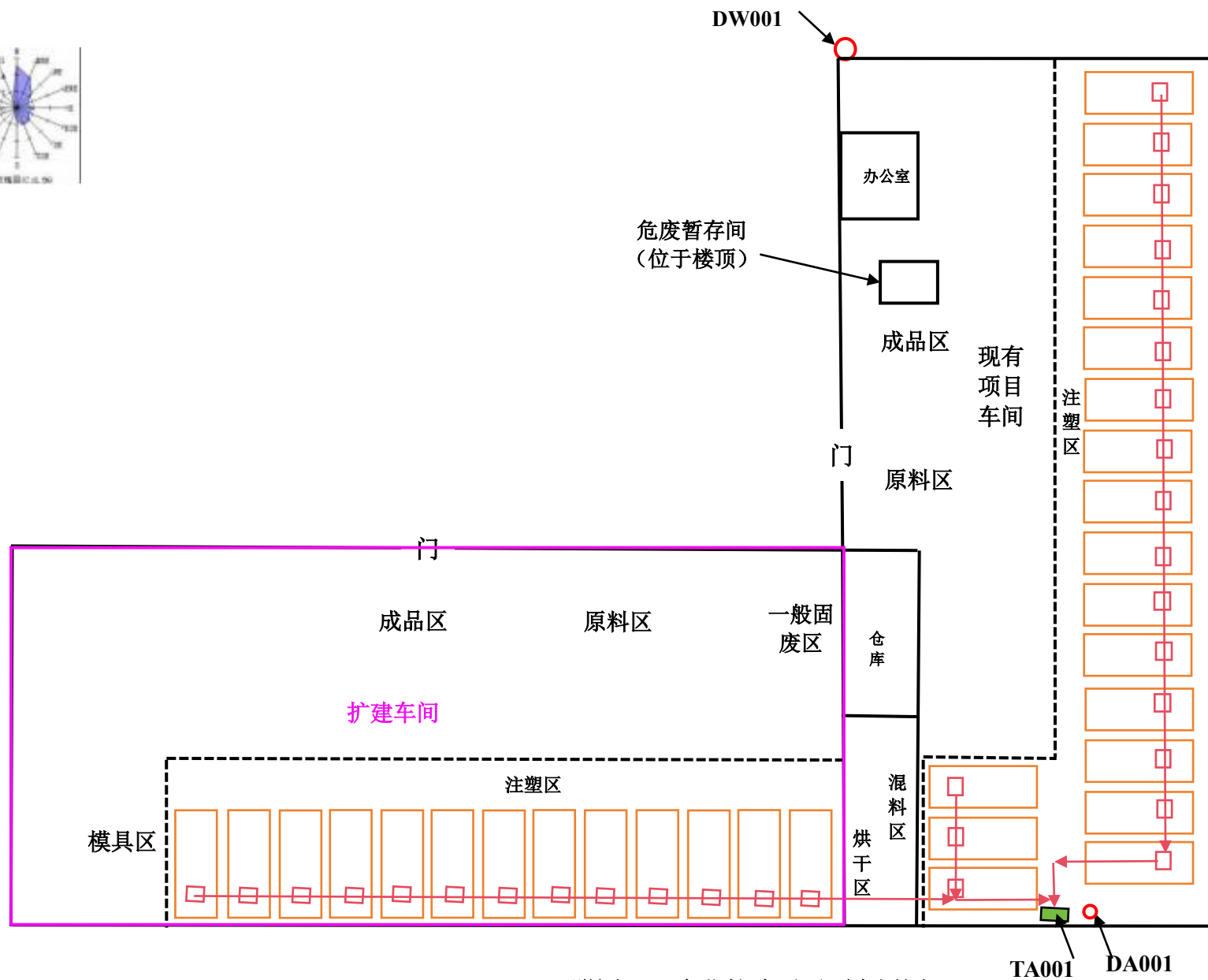
附图 4-2 企业扩建后平面布置图
