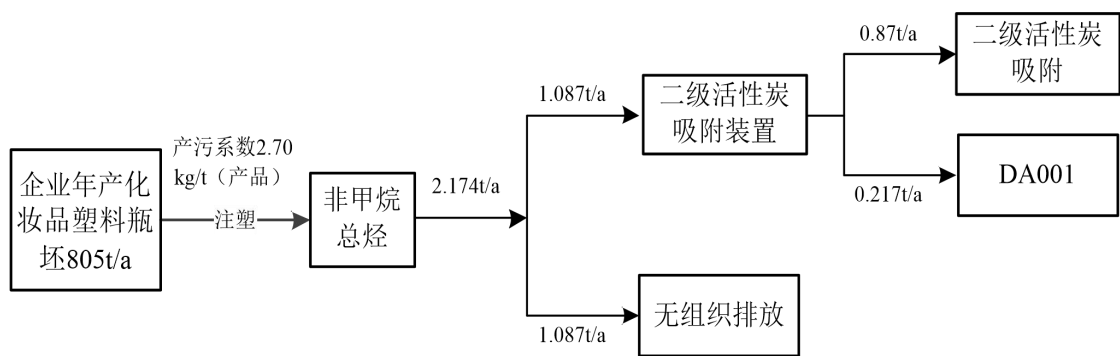
图 2-2 本项目 VOCs 平衡图
