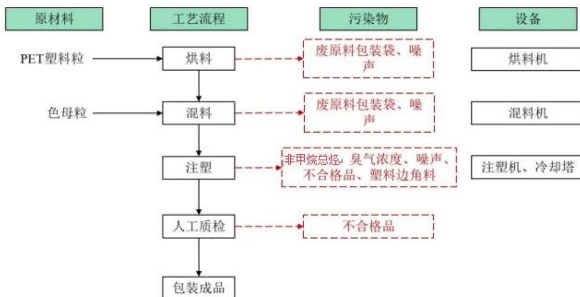
图 2-4 现有项目化妆品塑料瓶坯生产工艺流程及产污环节图
