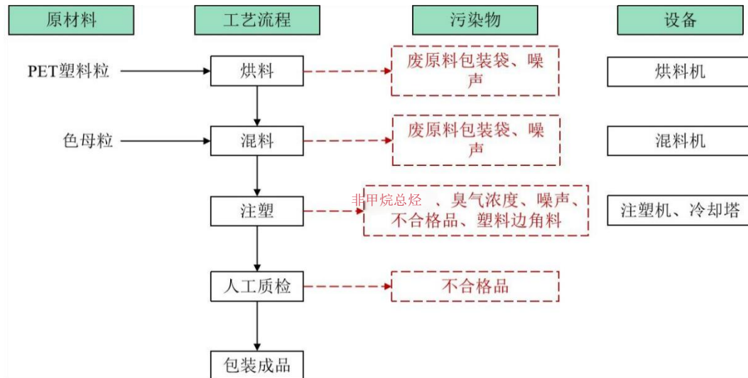
图 2-3 本项目化妆品塑料瓶坯生产工艺流程及产污环节图
