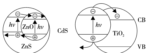
CB为半导体的导带；VB为半导体的价带；⊕为空穴；⊖为电子
