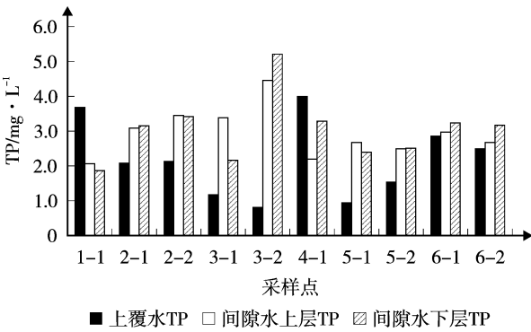
图 5 TP 浓度分布
