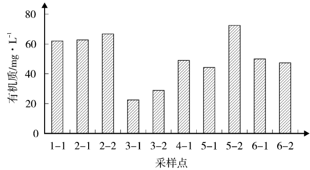
图 4 沉积物有机质平均含量分布
