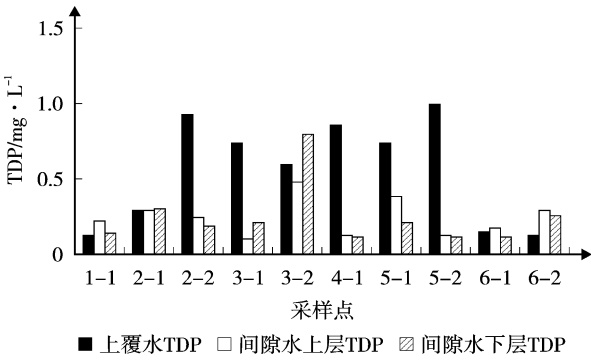
图 6 TDP 浓度分布
