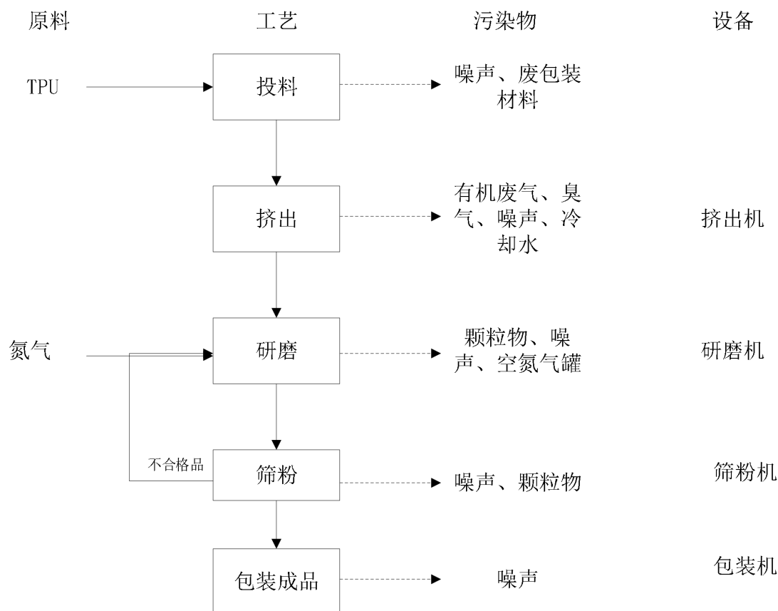
图 2-3 项目生产工艺流程图
