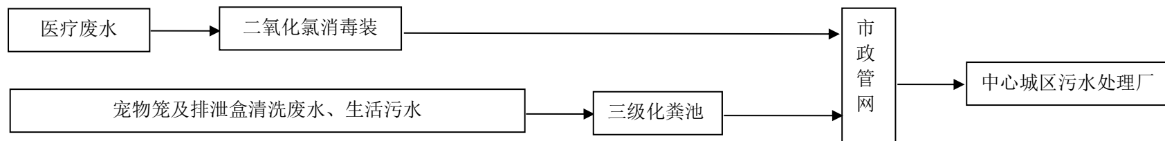
图 4-1 项目废水处理工艺流程图
