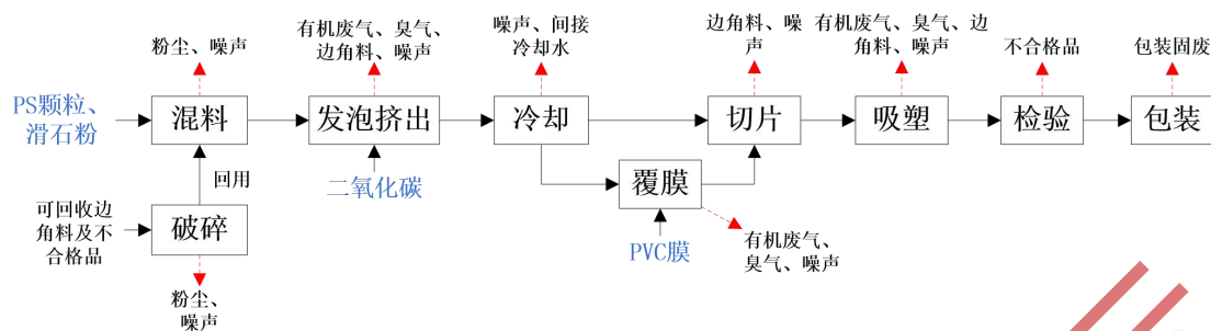
图 2-3 PS 泡沫托盘生产工艺流程及产污节点图
