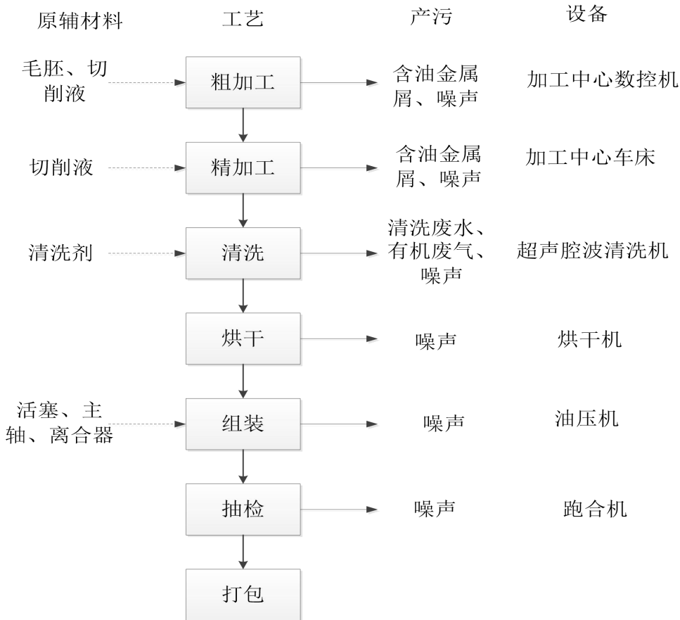
图 2-2 项目毛胚的加工及空调压缩机的组装工艺流程
