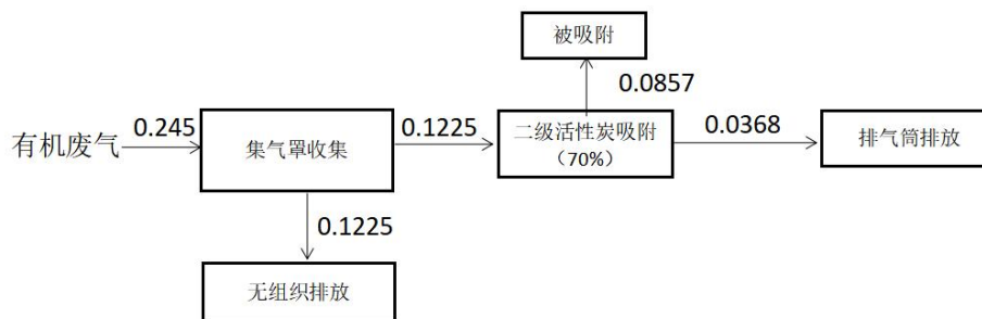
图 4-1 项目有机废气平衡图 (t/a)
