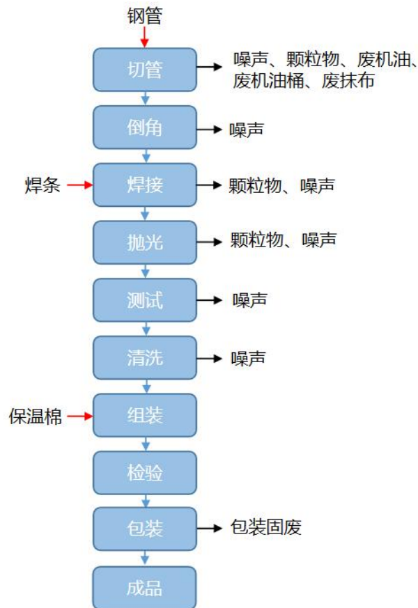
图2-3 液冷总成生产工艺流程图
