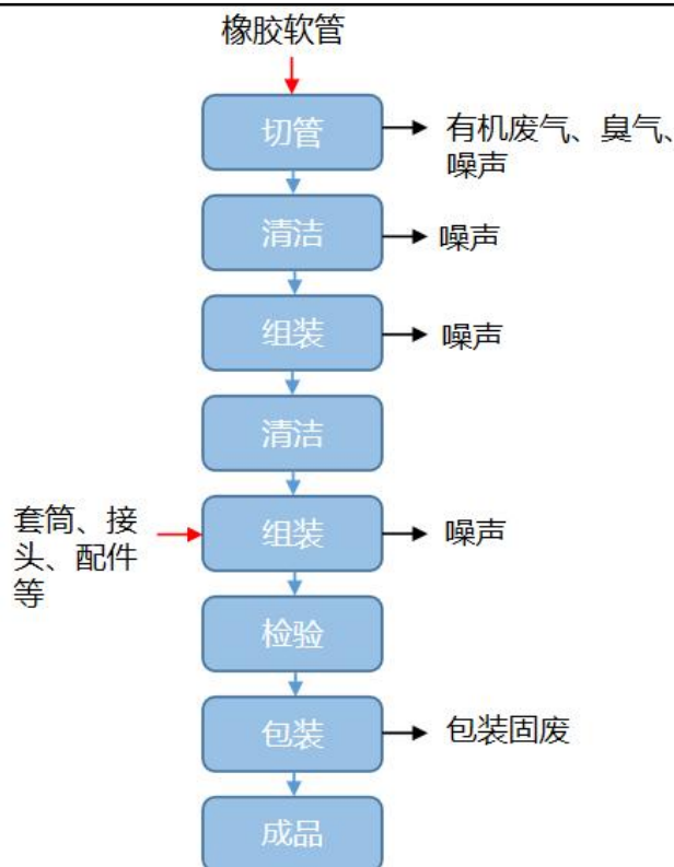
图2-2 软管总成生产工艺流程图
