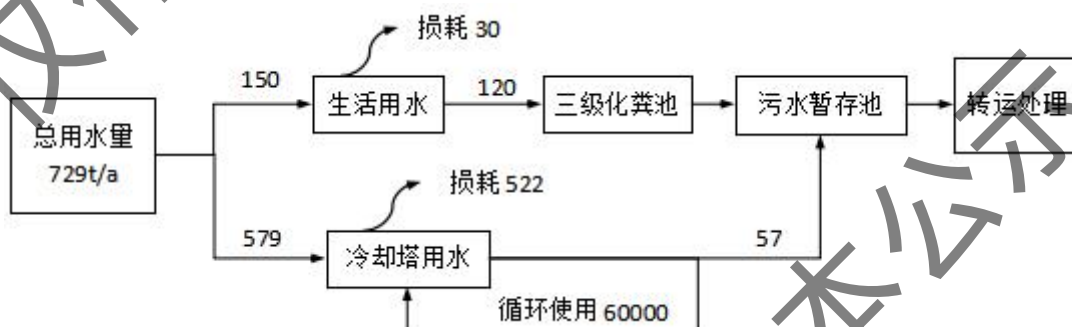
图 2-1 近期项目水平衡图 (t/a)
