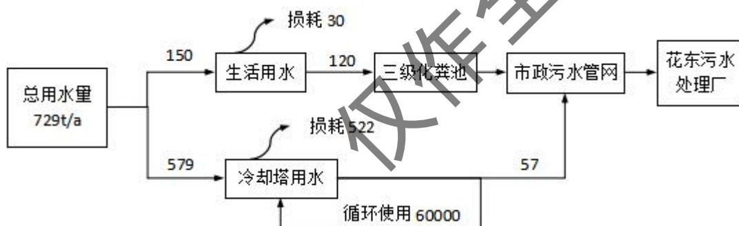
图 2-2 远期项目水平衡图 (t/a)
