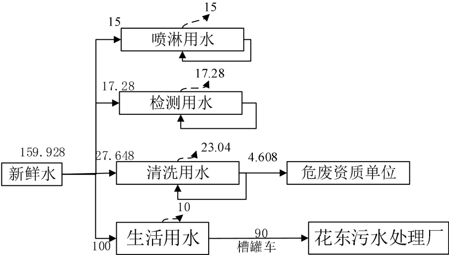
图 2-1 项目近期水平衡图（单位：t/a）
