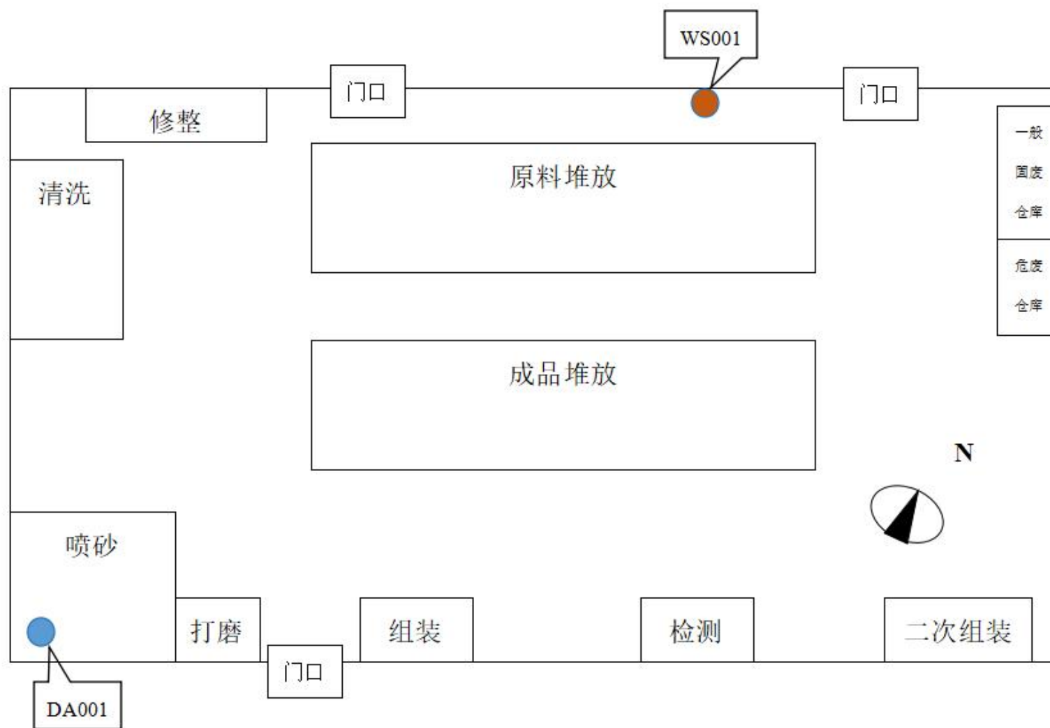
附图 5 项目厂区总平面布置图
