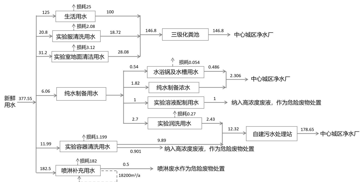
图2 本项目水平衡图 单位: t/a
