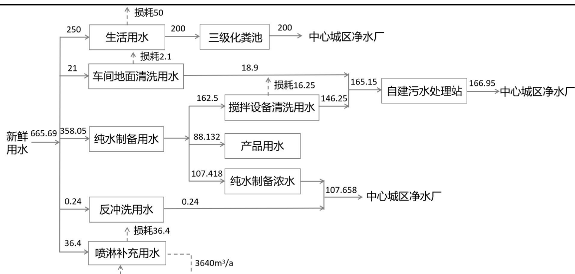
图1 现有项目水平衡图 单位: t/a
