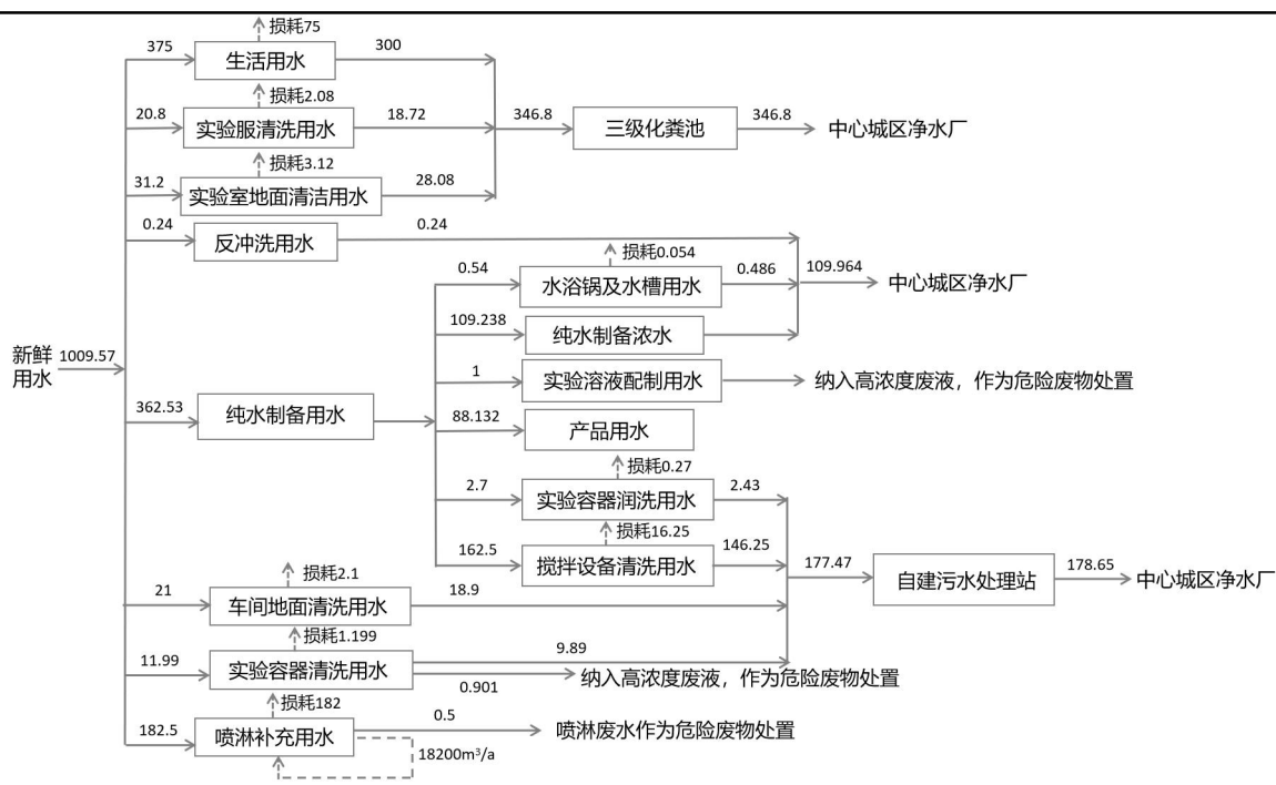
图3 扩建后项目水平衡图 单位: t/a
