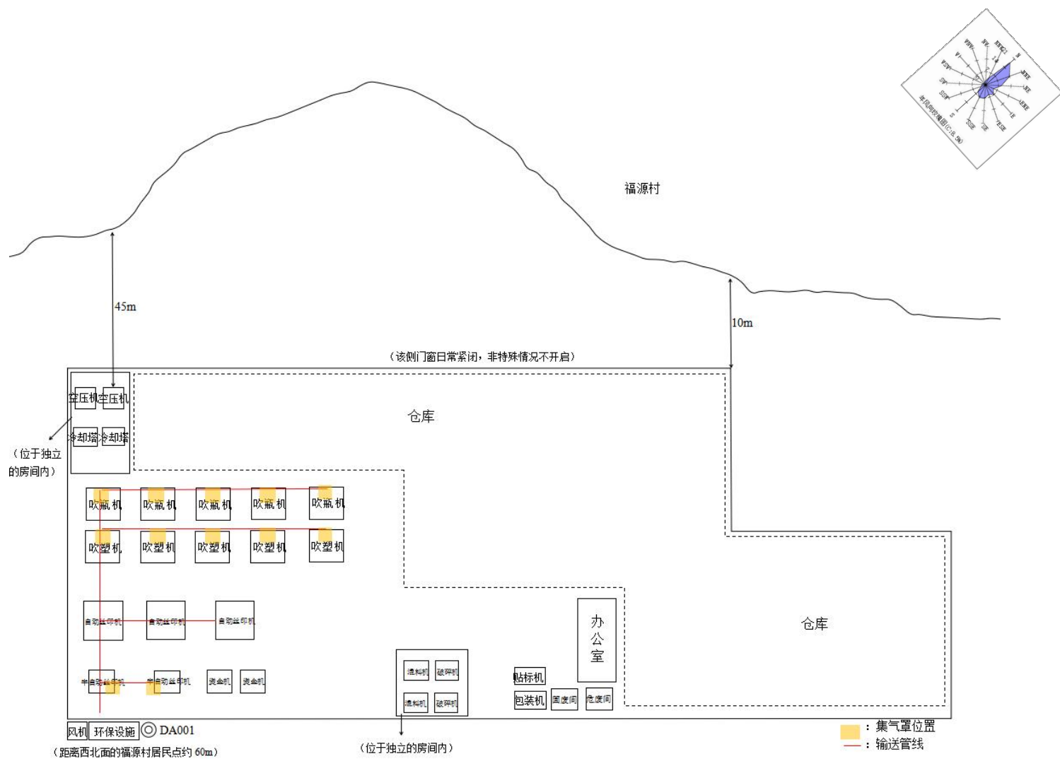
附图 5 项目平面布置图
