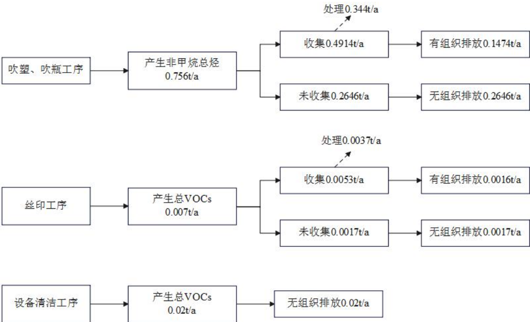
图 4-1 项目 VOCs 平衡图
