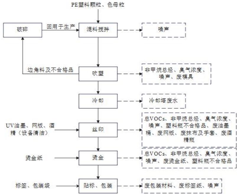
图 2-2 PE 塑料瓶生产工艺流程及产污图
