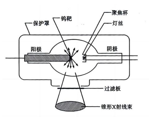
图 9-2 X 射线管示意图
