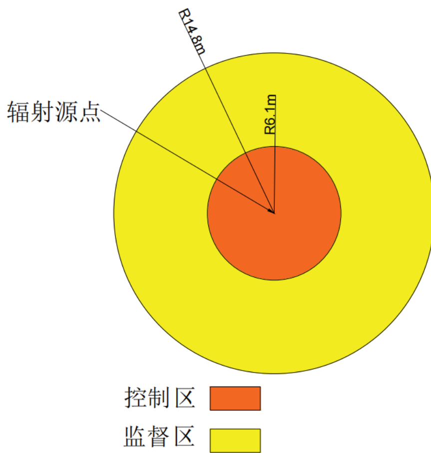
图 10-2 垂直向上照射时监督区和控制区范围示意图
