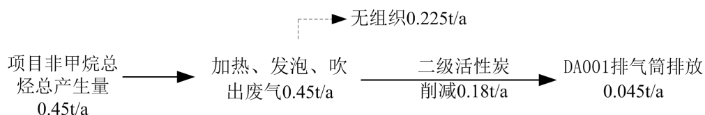
图 4-1 项目有机废气平衡图
