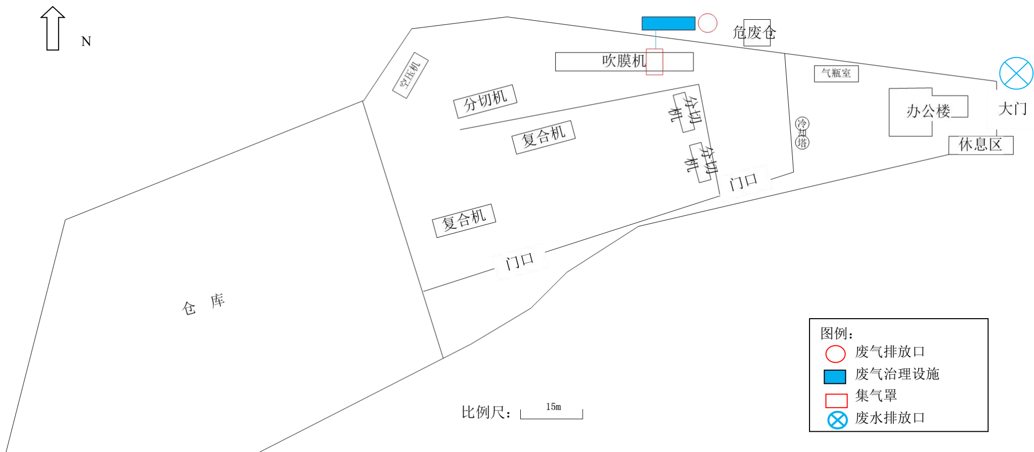
附图 5 建设项目生产车间平面布置图
