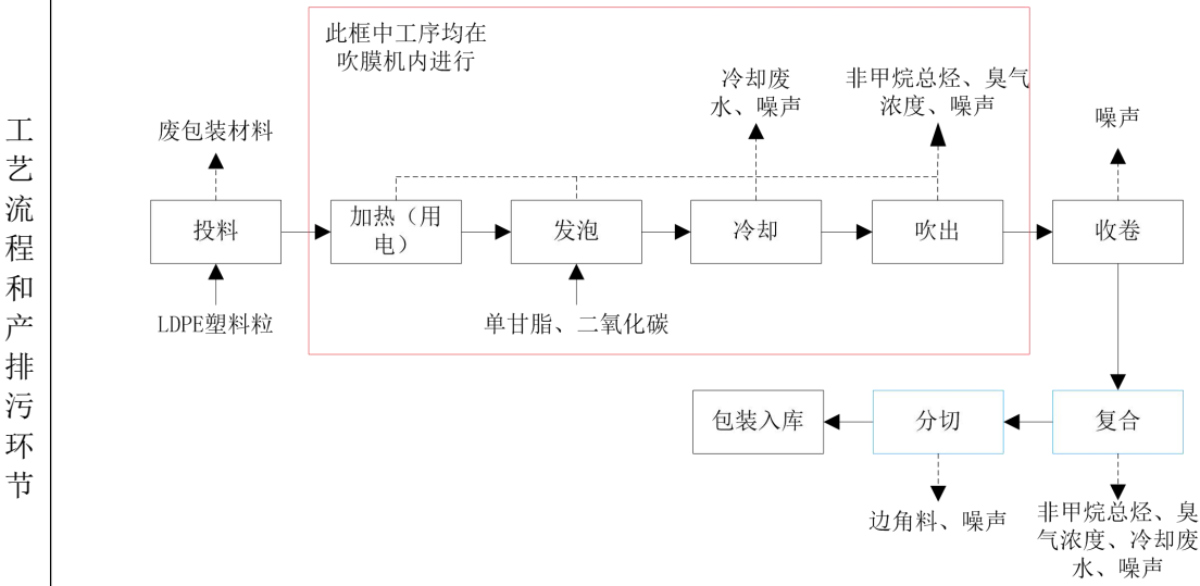
图 2-2 产品生产工艺流程图
