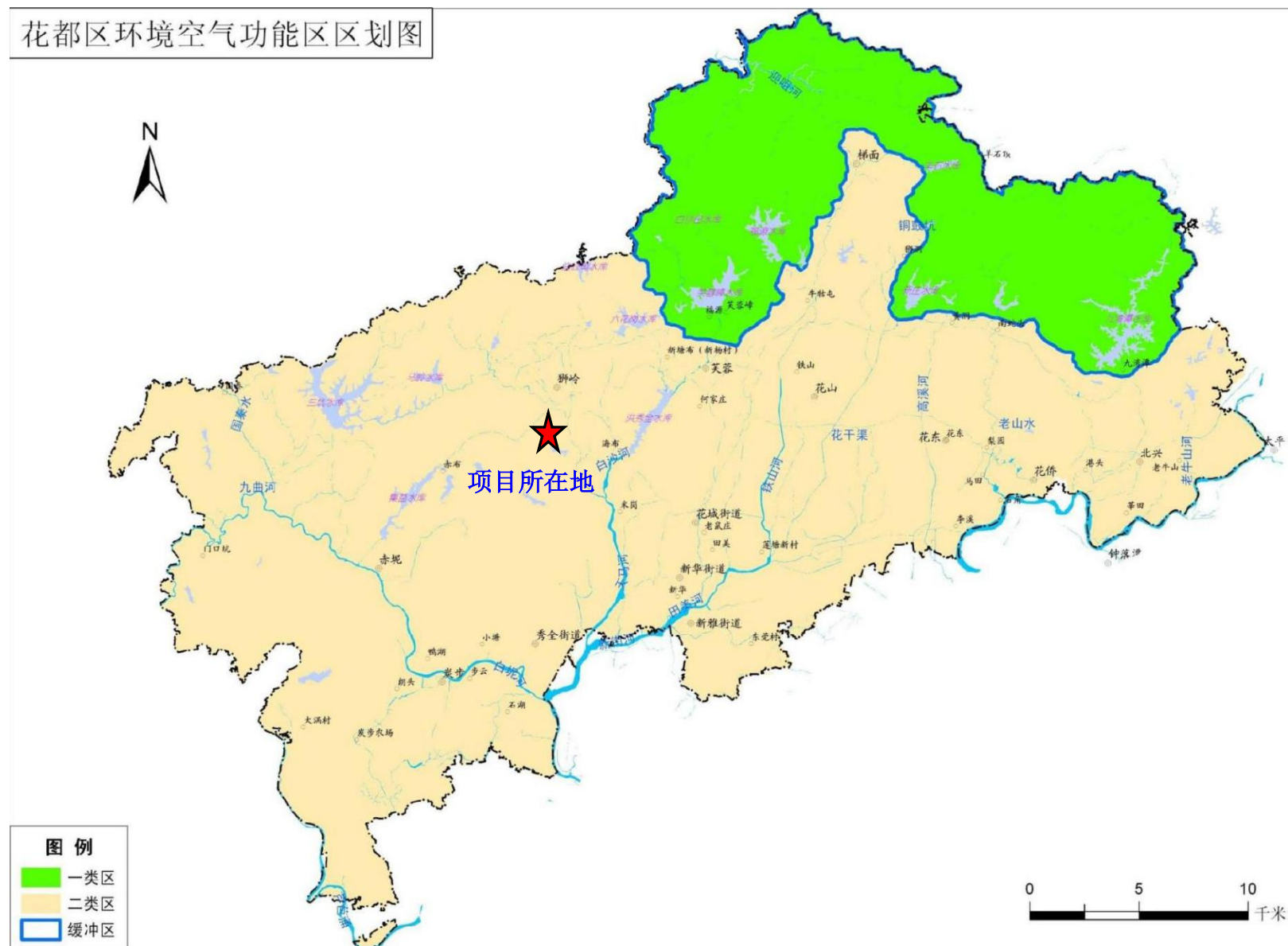
附图 7 广州市花都区环境空气功能区划图
