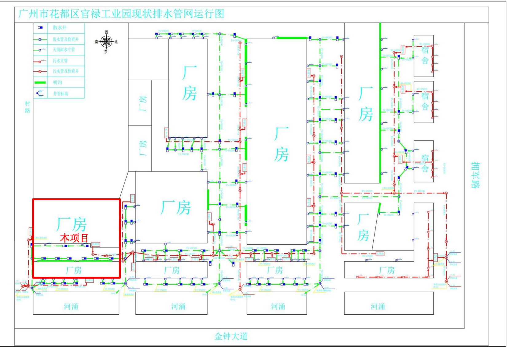
附图 19 官禄工业园排水管网图
