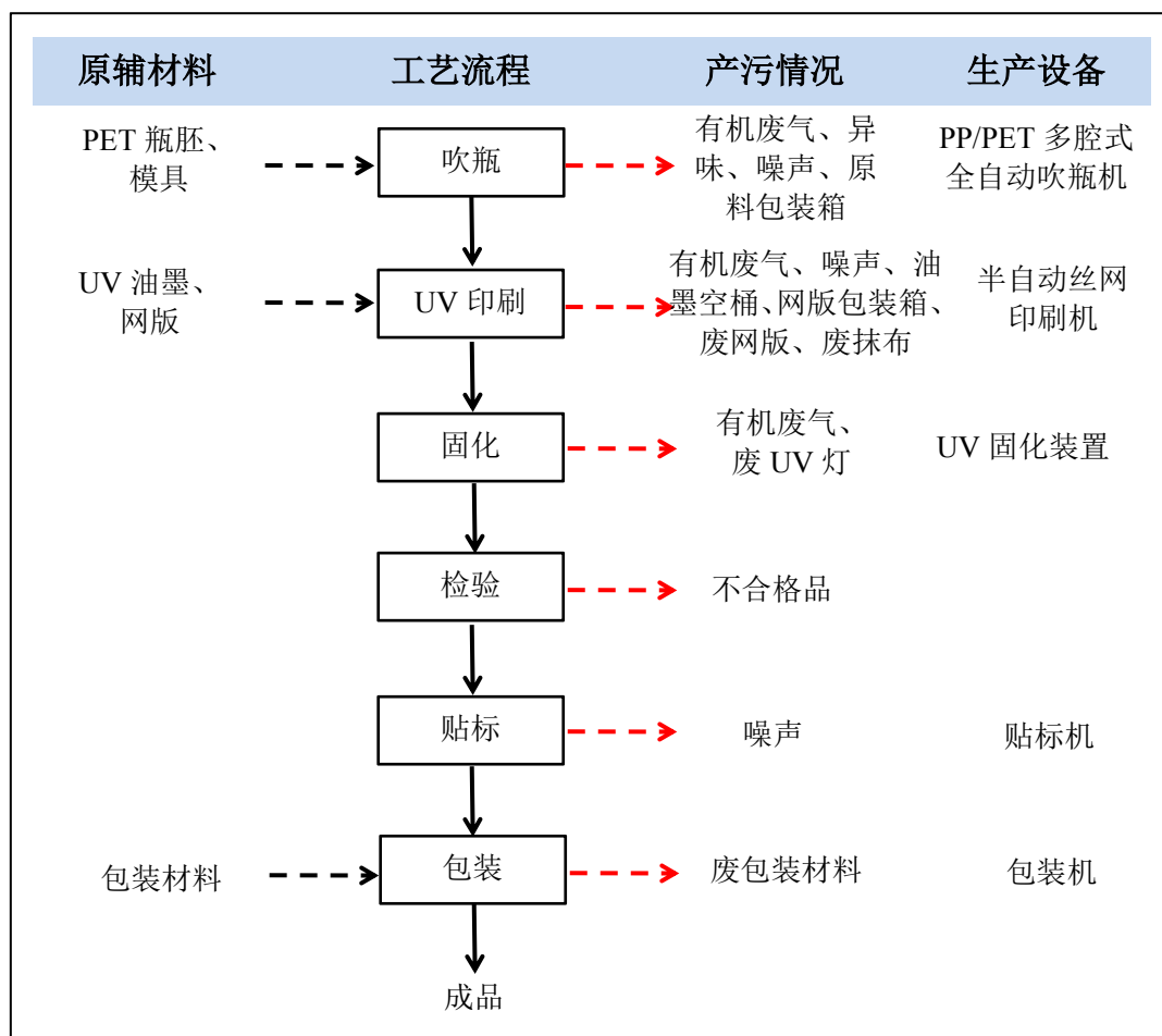
图 2-3 PET 塑料瓶生产工艺及产污情况图
