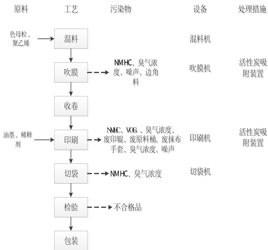
图 2-2 项目生产工艺流程图
