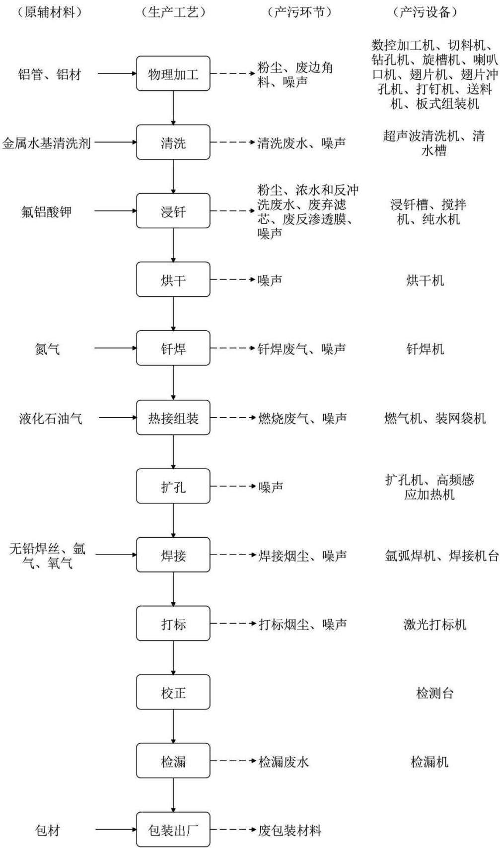
图 2-3 汽车水箱油冷器（铝制品）生产工艺流程与产污环节示意图
