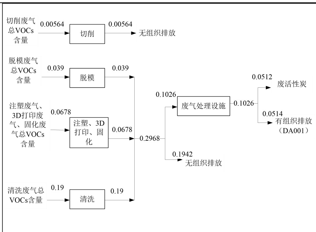
图 4-1 VOCs 平衡图
