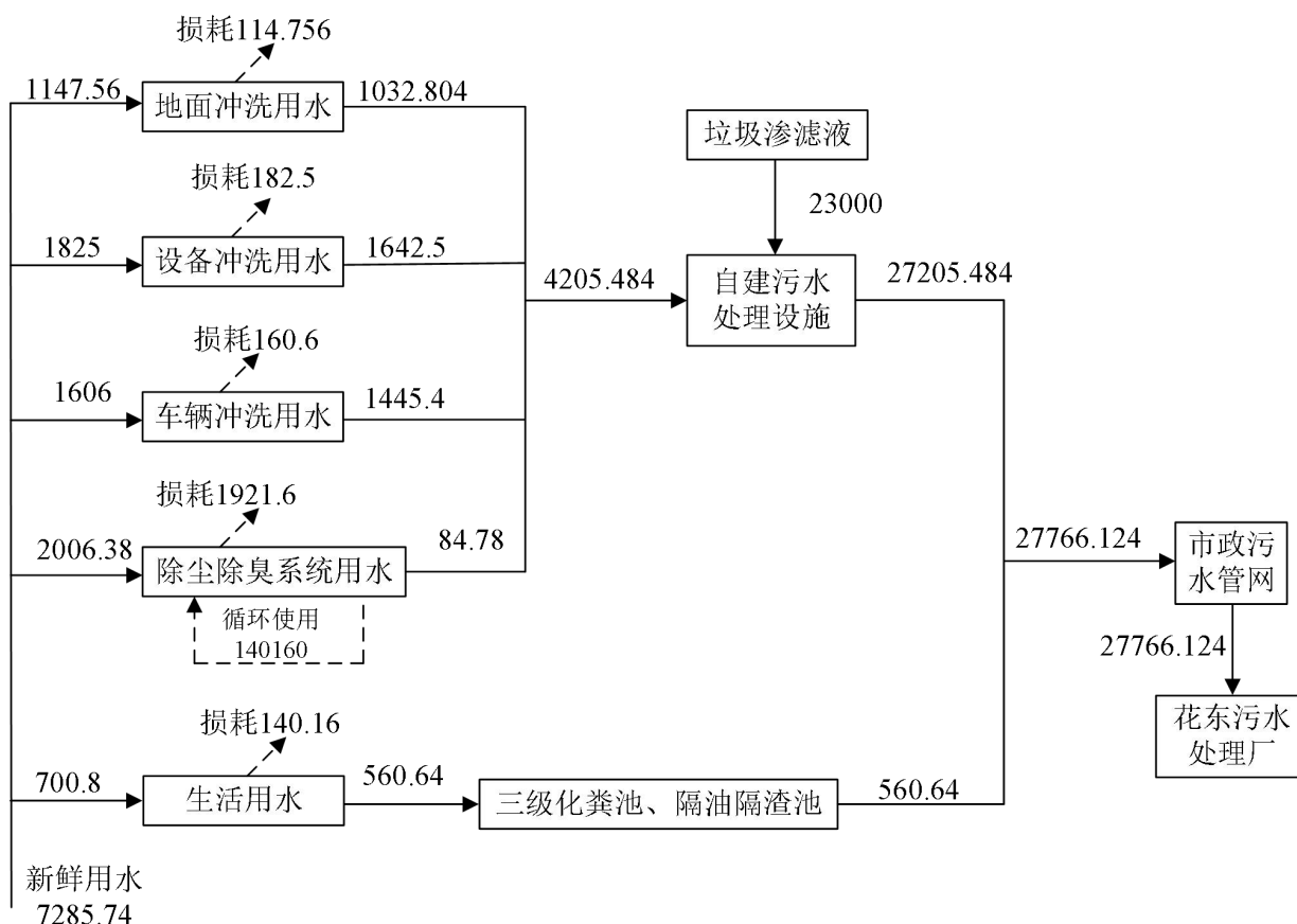
图 2-1 (b) 项目 1000t/d 处理规模的水平衡图 (单位: m³/a)
