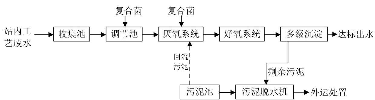
图 4-1 项目自建污水处理设施工艺流程图
