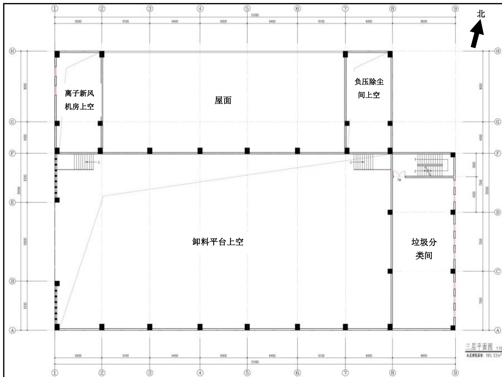
附图 5-4 压缩车间三层平面图
