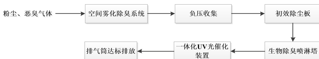
图 4-8 废气处理工艺示意图
