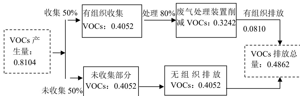
图 2-1 VOCs 平衡图 (t/a)
