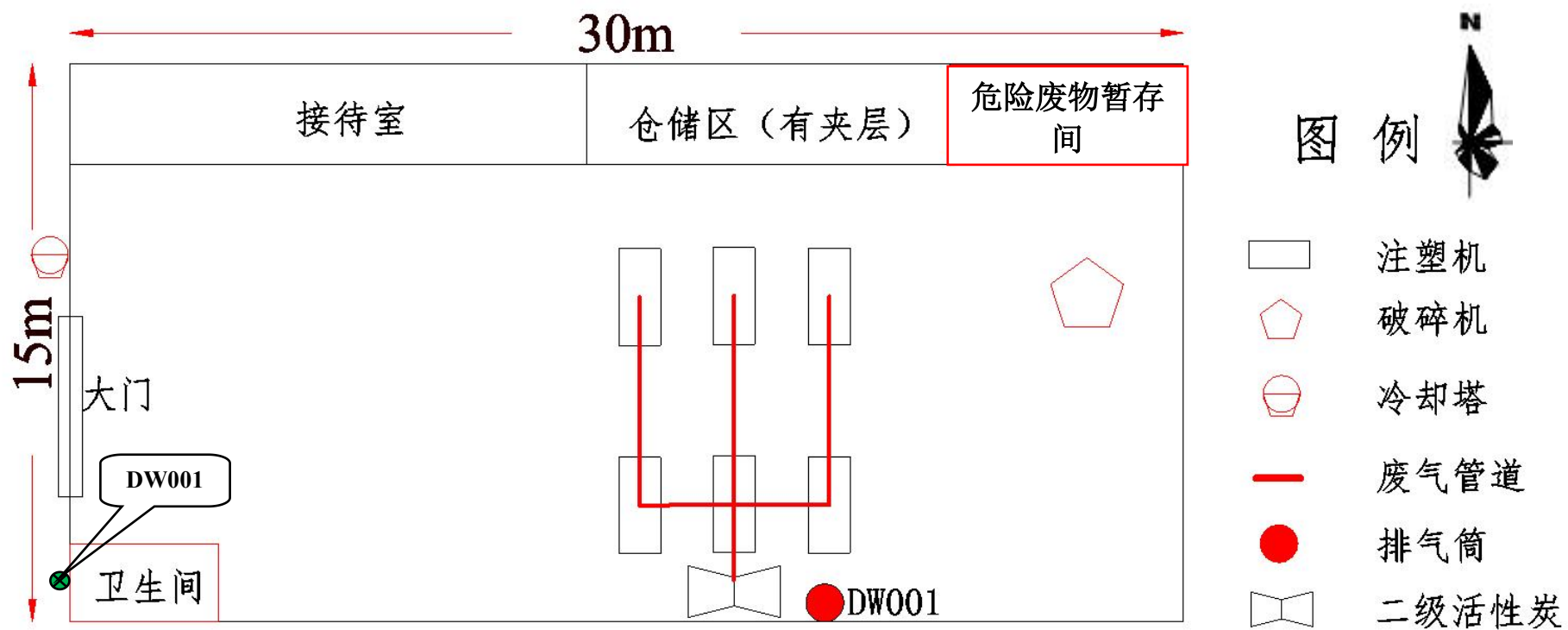
附图 4 本项目总平面布置图
