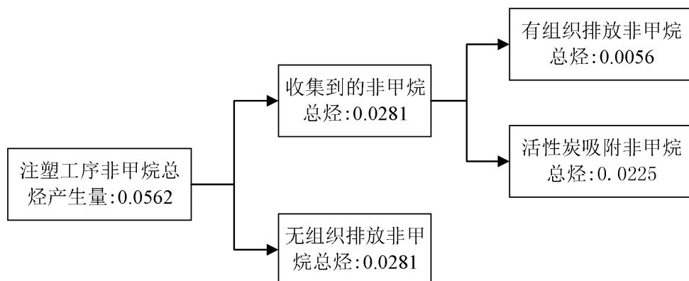
图 4-1 本项目非甲烷总烃平衡图 (t/a)
