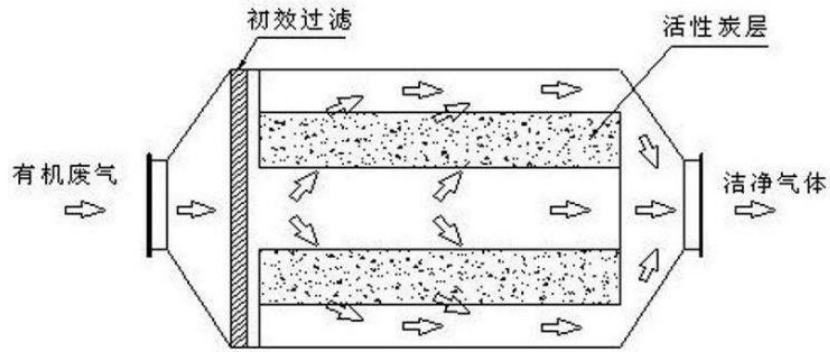
图 4-3 活性炭箱示意图
