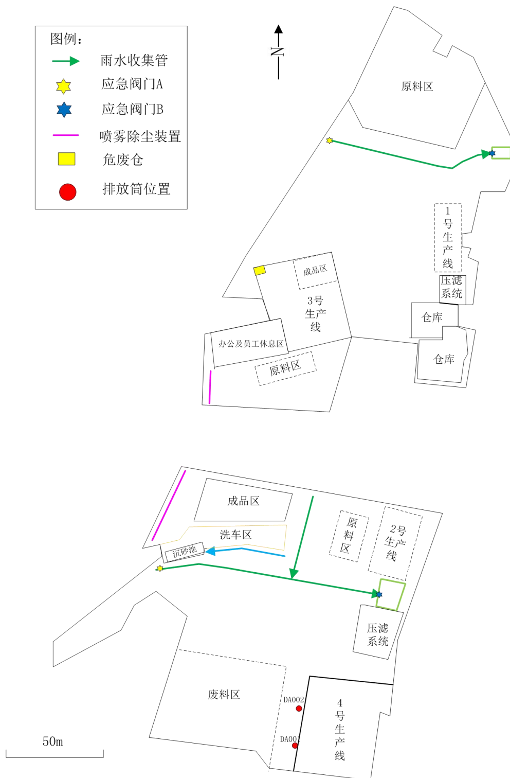
附图5 项目总平面布置图
