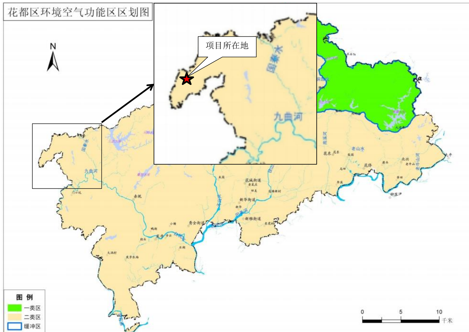
附图 12 项目环境空气质量功能区划图
