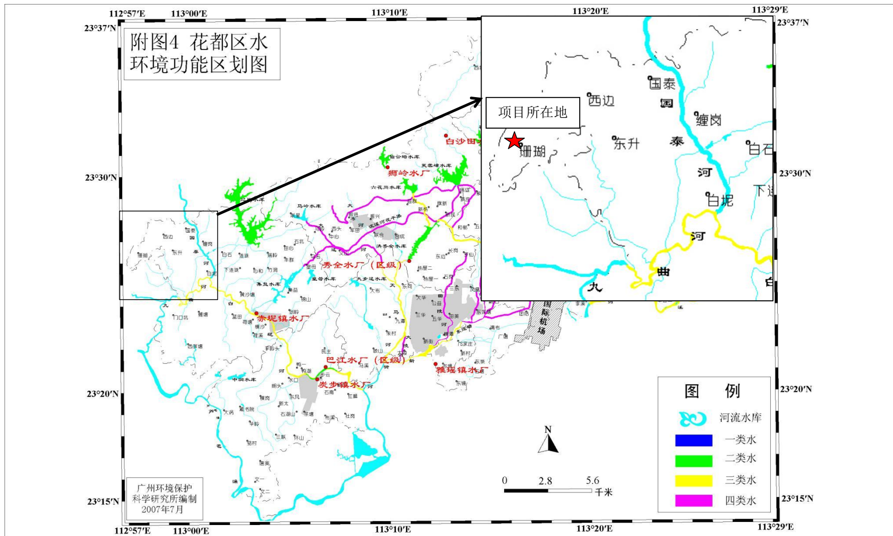
附图9 项目地表水环境功能区划图
