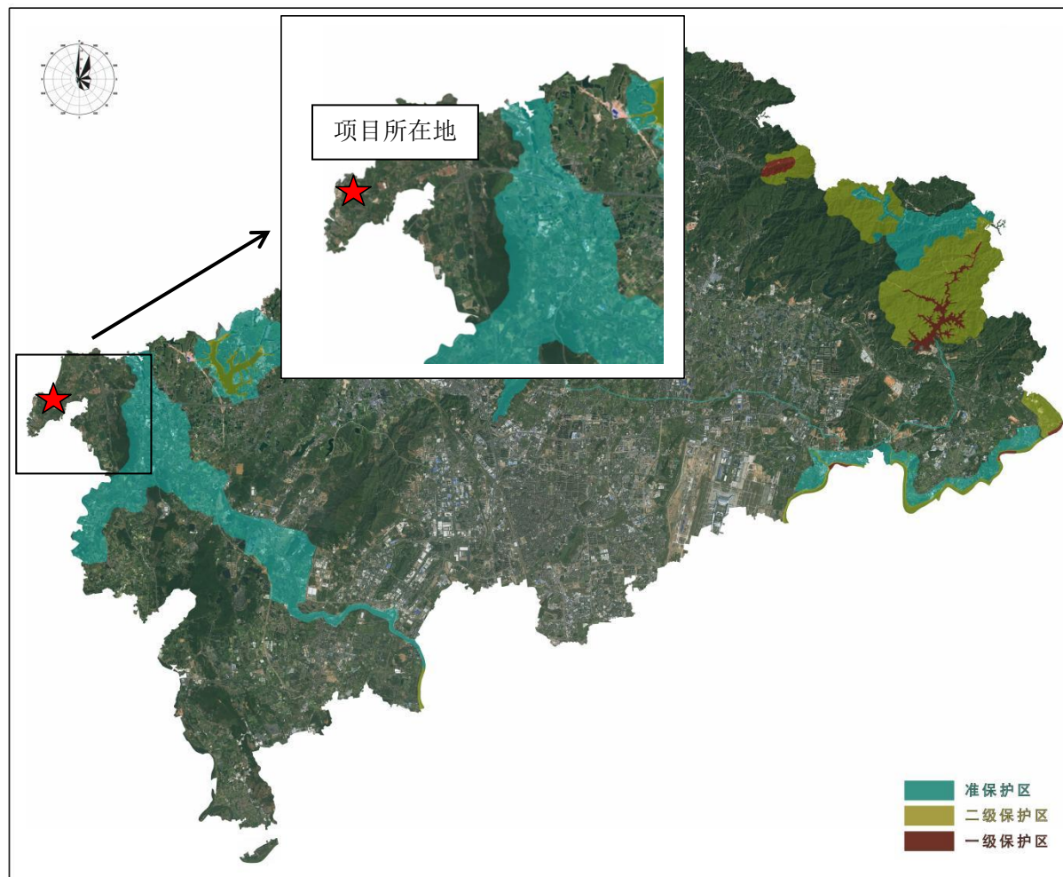
附图 10 项目饮用水源保护区划图
