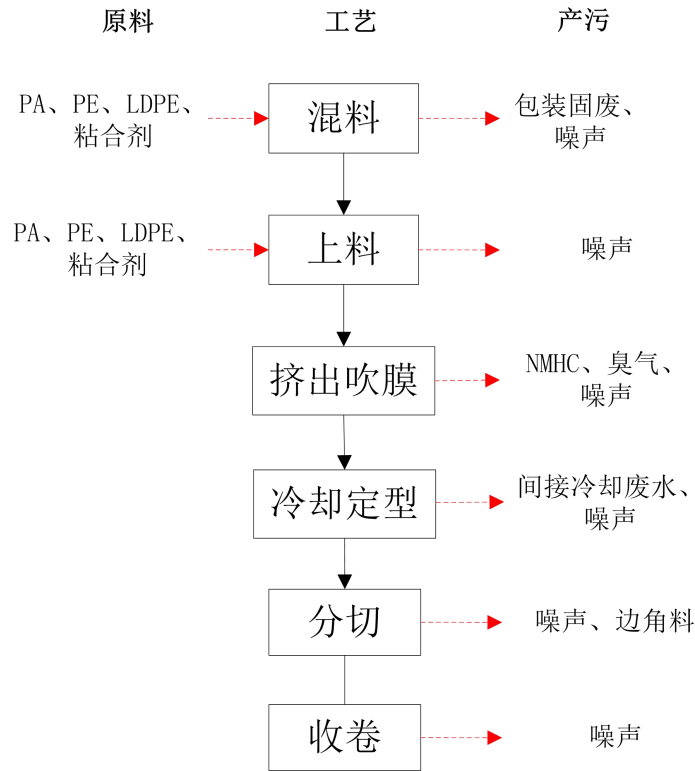
图 2-2 尼龙共挤膜生产工艺及产排污环节图
