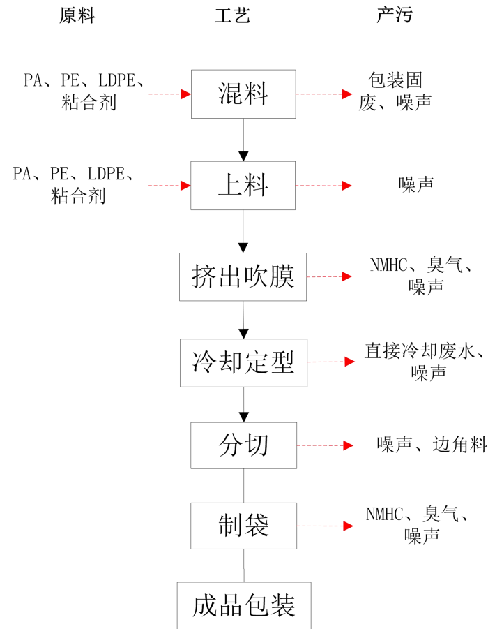
图 2-3 真空袋生产工艺及产污环节图
