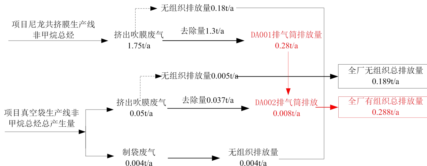
图4-1 全厂有机废气平衡图
