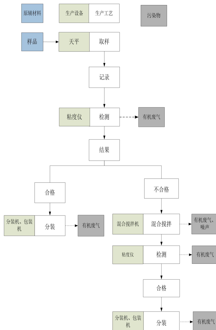
图2-9品检室生产工艺流程图
