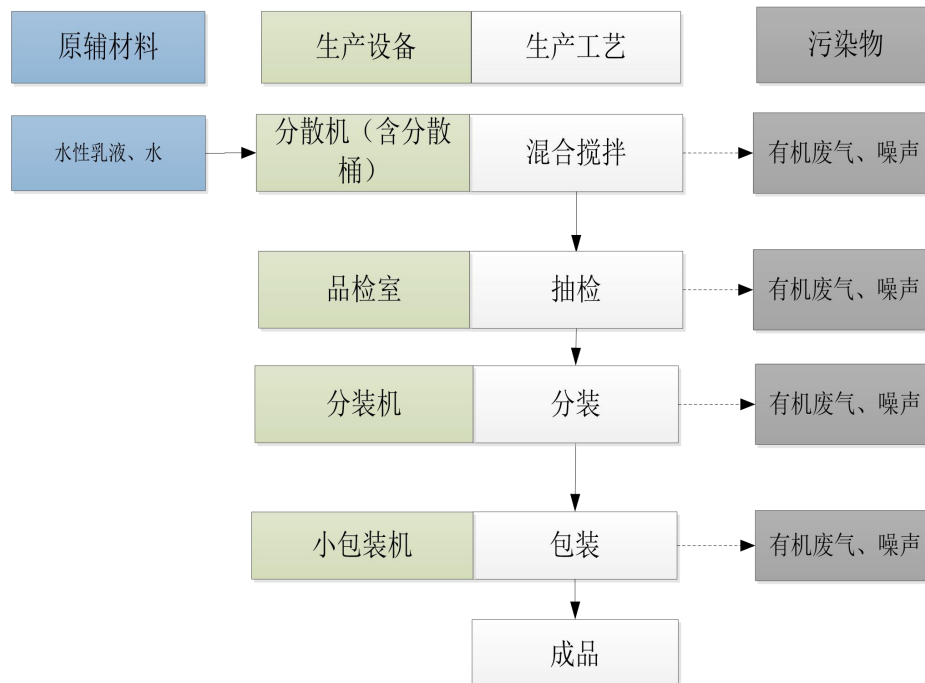
图2-6界面剂产品生产工艺流程图
