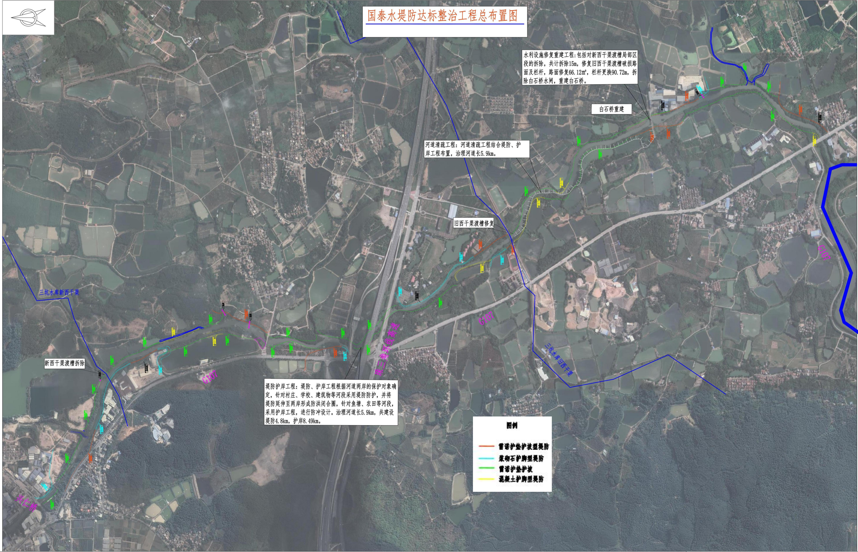
附图 3 项目工程总布置图
