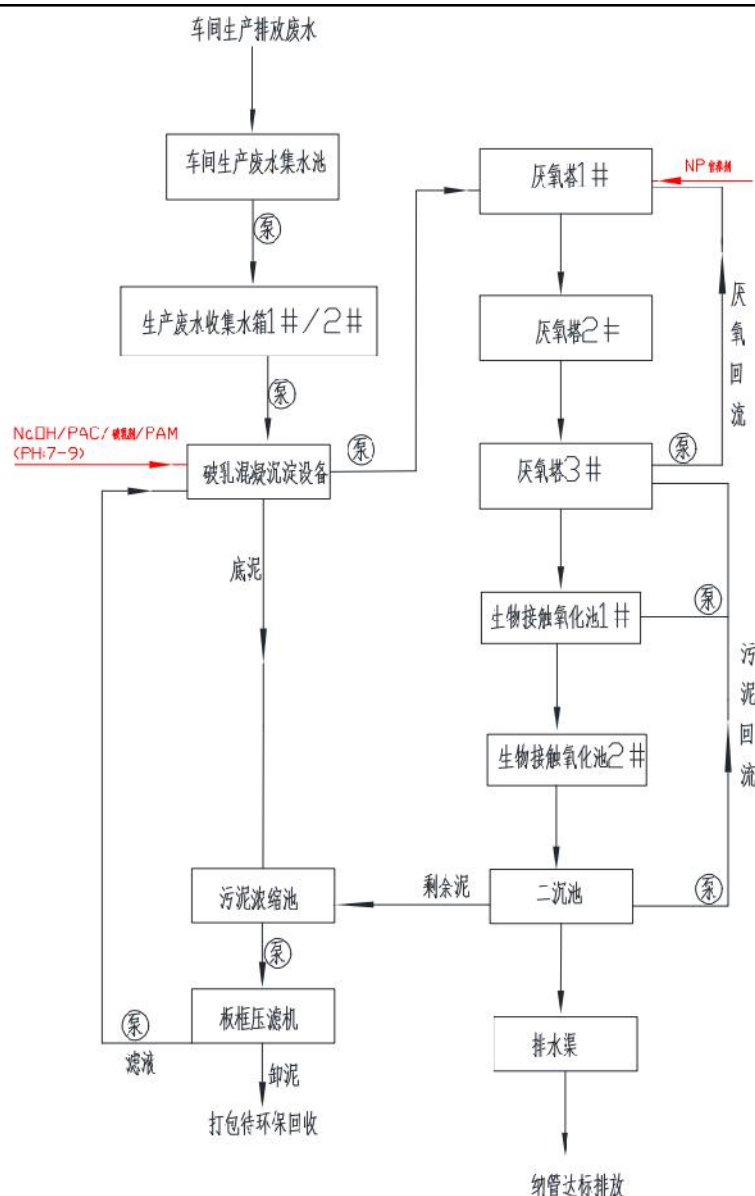
图 4-1 自建污水处理站工艺流程图
