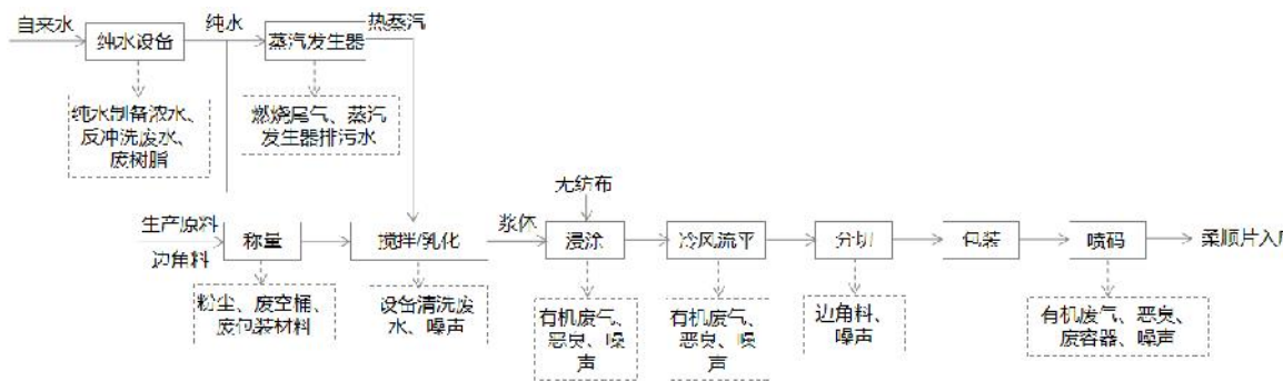
图 2-3 迁建后柔顺片生产工艺流程图
