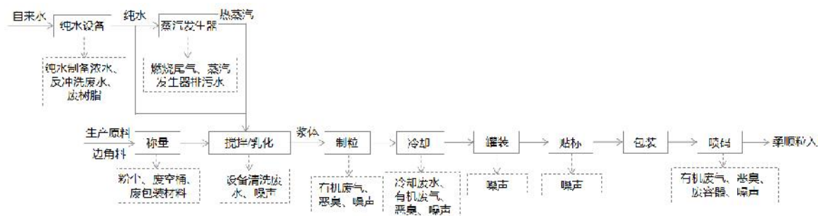
图 2-4 迁建后柔顺粒生产工艺流程图
