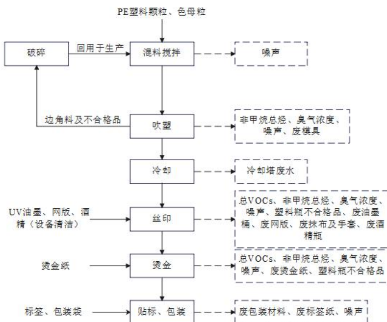
图 2-2 PE 塑料瓶生产工艺流程及产污图
