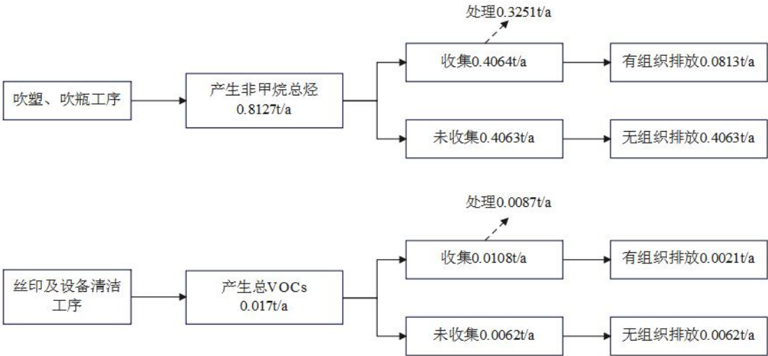
图 4-1 项目 VOCs 平衡图
