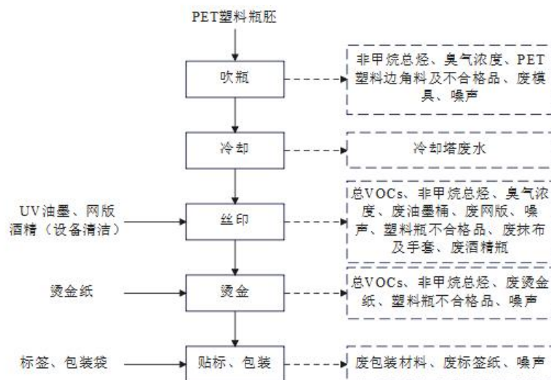
图 2-3 PET 塑料瓶生产工艺流程及产污图
