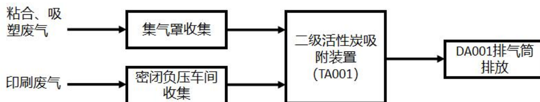
图 4-2 有机废气处理工艺
