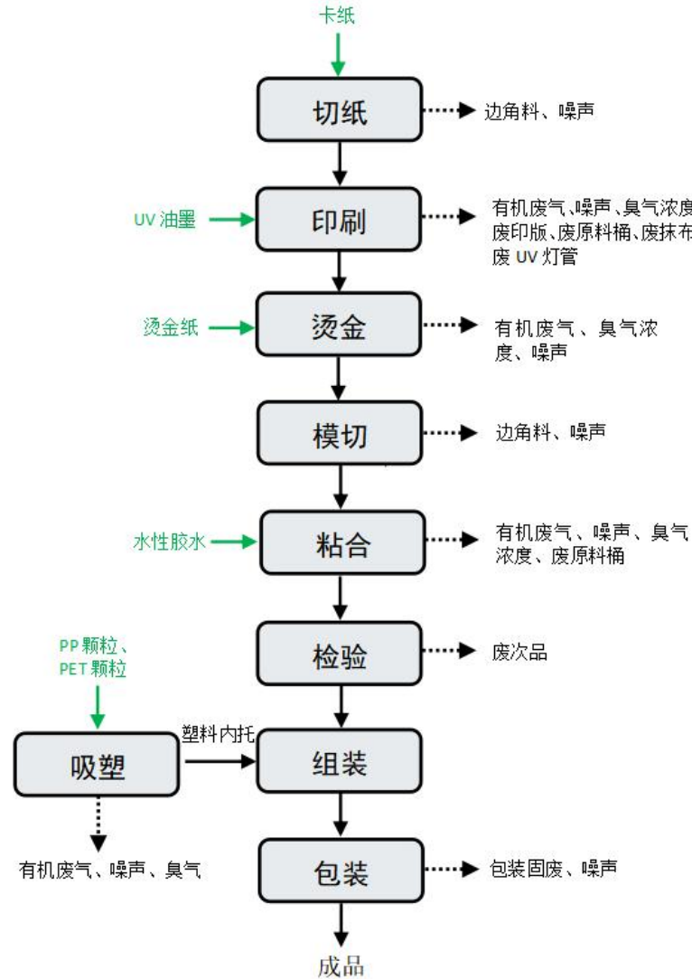
图 2-2 精装盒生产工艺流程图及产污环节
