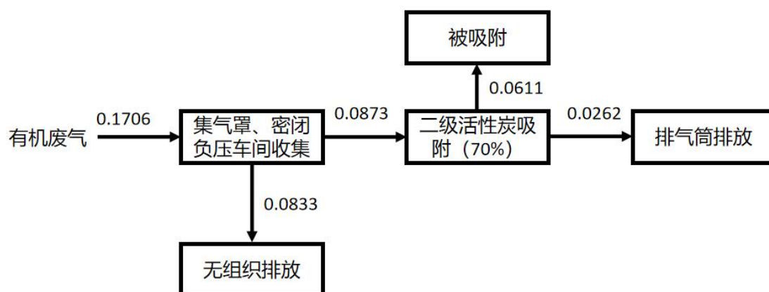
图 4-1 本项目有机废气平衡图（单位：t/a）
