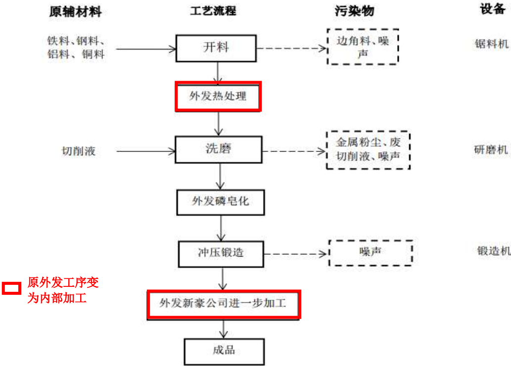
图 2-4 五厂（锻造件）工艺流程及产污环节图
