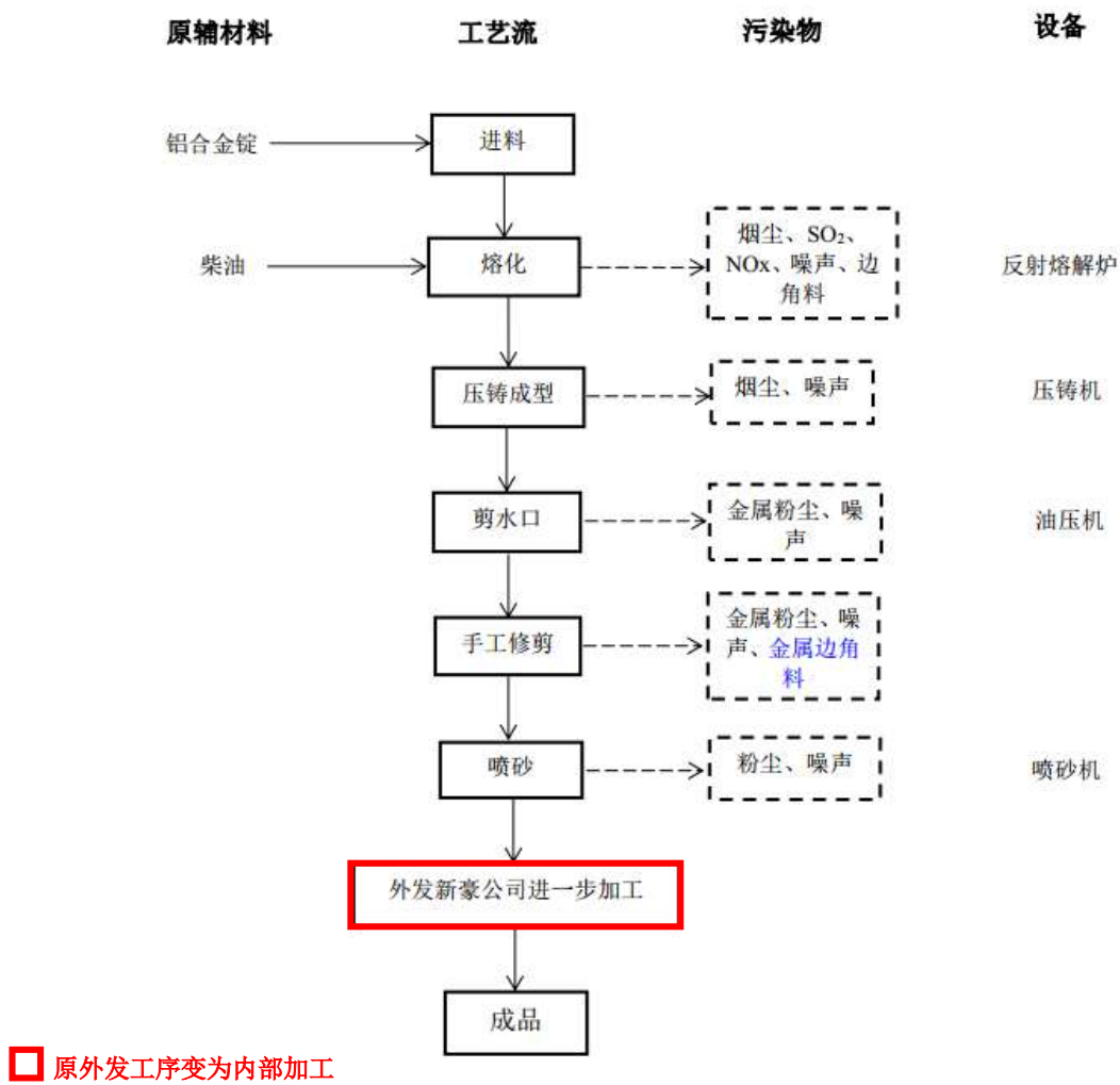
图 2-3 五厂（压铸件）工艺流程及产污环节图
