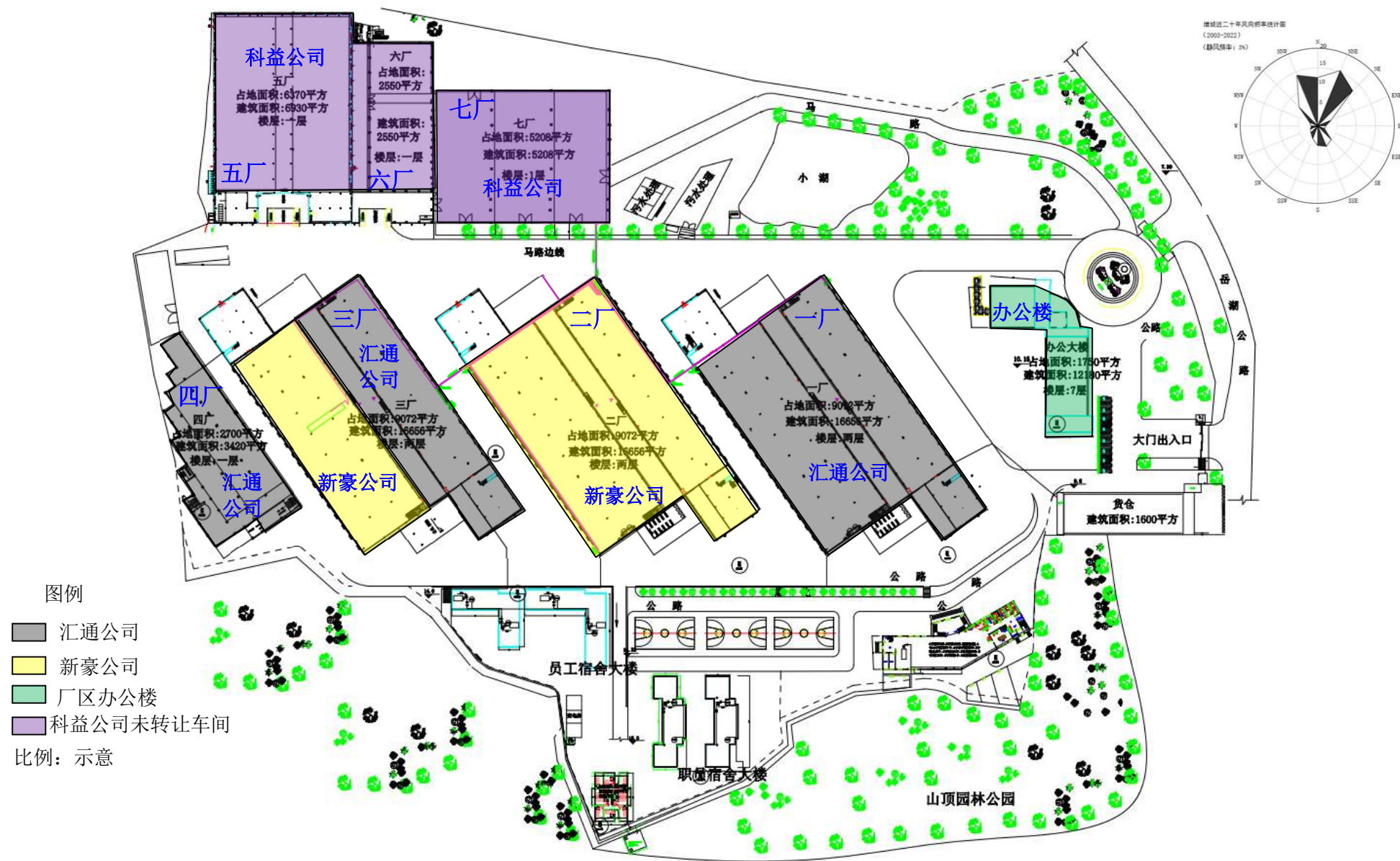
附图 3 建设项目平面布局图
