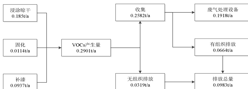
图 4-2 扩建项目 TVOC 平衡图
