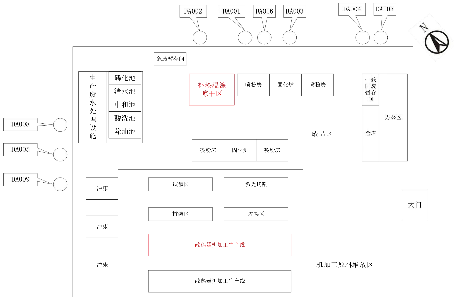
附图 4-2 现有项目 1#车间平面布置图（标红为扩建项目建设内容）
