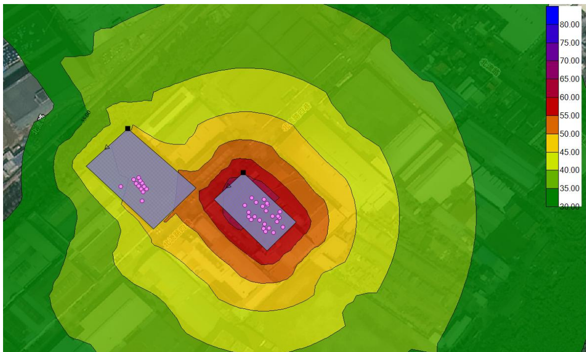
图 4-6 计算结果等值线图
