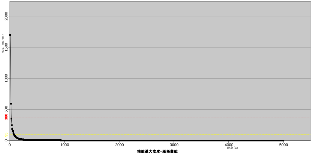
图 5.1-4 最不利气象条件下 CO 最大浓度值与距离曲线图
