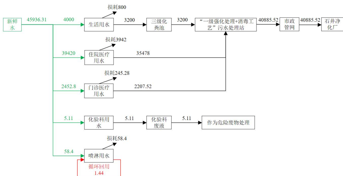
图 2-4 项目扩建后年水平衡图 (单位: \text{m}^3/\text{a} )
