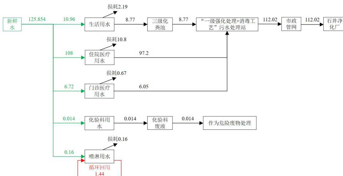
图 2-3 项目扩建后日水平衡图 (单位: \text{m}^3/\text{d} )
