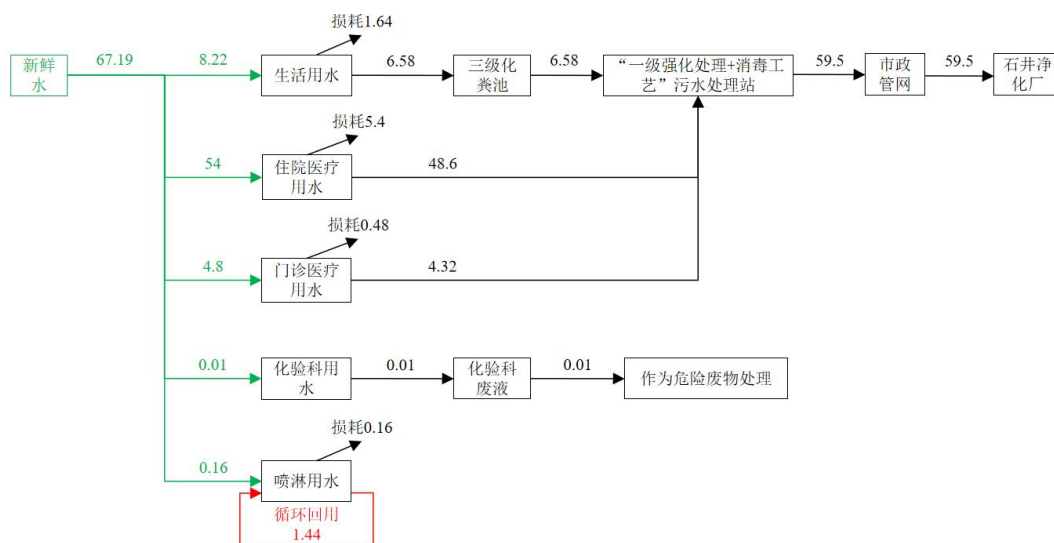
图 2-1 现有项目日水平衡图 (单位: \text{m}^3/\text{d} )
