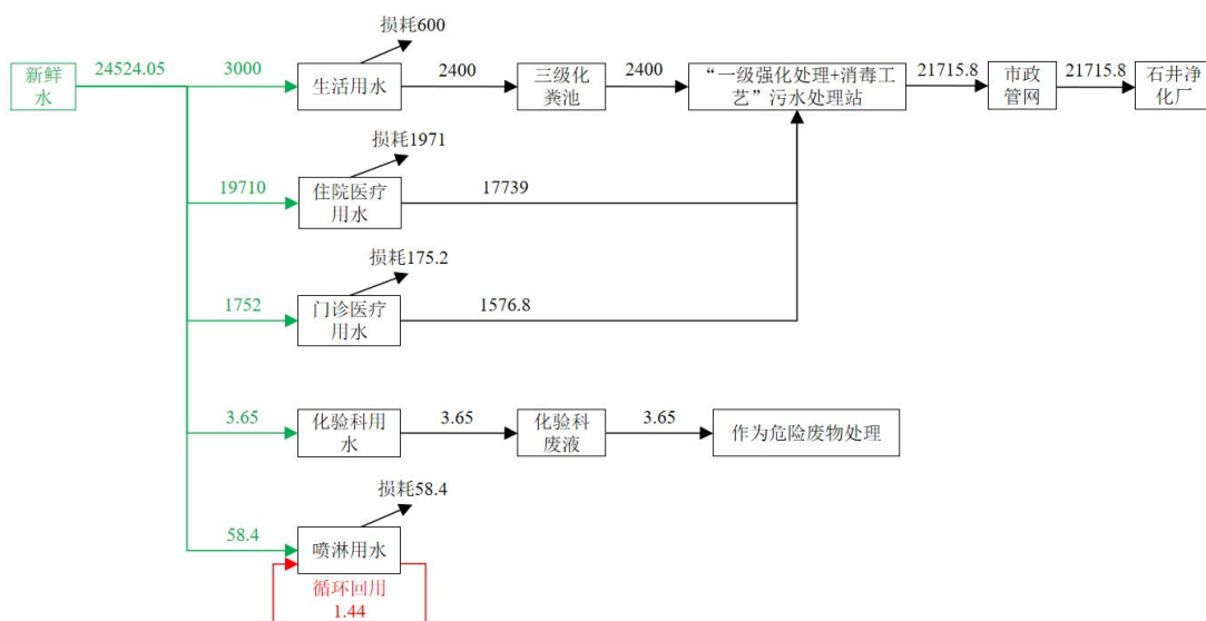
图 2-2 现有项目年水平衡图 (单位: \text{m}^3/\text{a} )
